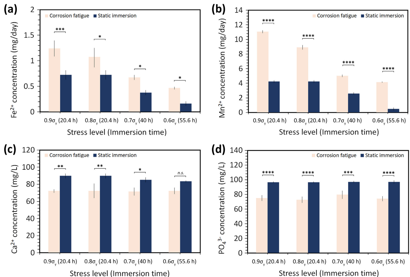
Fig. 3. (a) \text{Fe}^{2+} , (b) \text{Mn}^{2+} , (c) \text{Ca}^{2+} , and (d) \text{PO}_4^{3-} ion concentrations in r-SBF after the corrosion fatigue tests.
