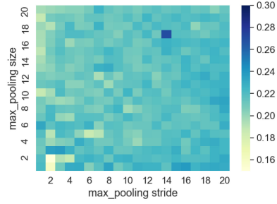
(d) ACC : tuning the last max-pooling layer (min: 0.149; max: 0.270)
