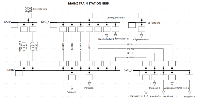
Fig. 2. Mainz Hauptbahnhof Grid
