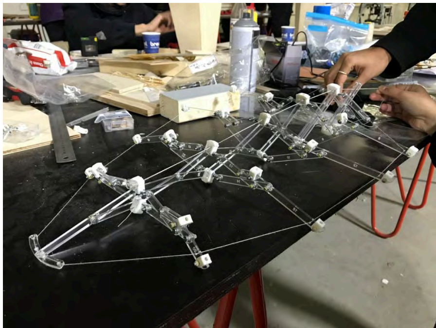
Fig.5 functiemodel van een zonluifel 1:5 (door Kritika Agarwal, Priyadarshini Nanda, Shweta Kamble, Pierre Kauter en Okan Türkan, gebruik met toestemming).
