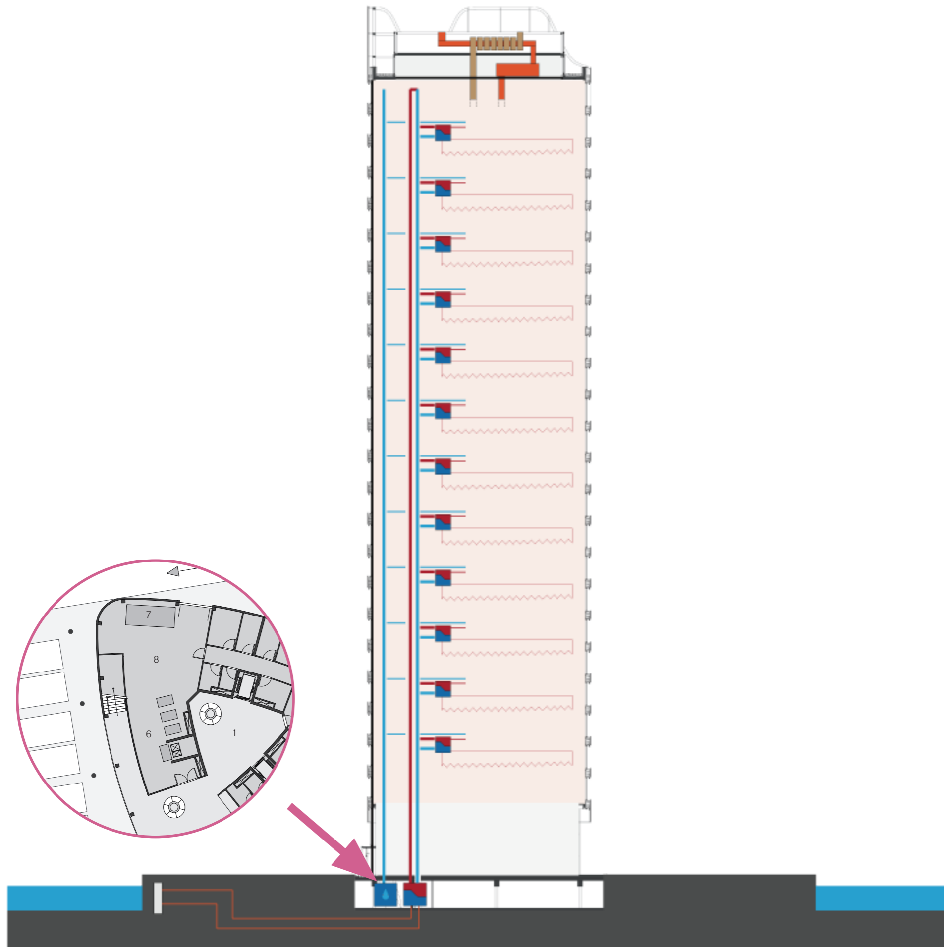
klimatiserings principe
