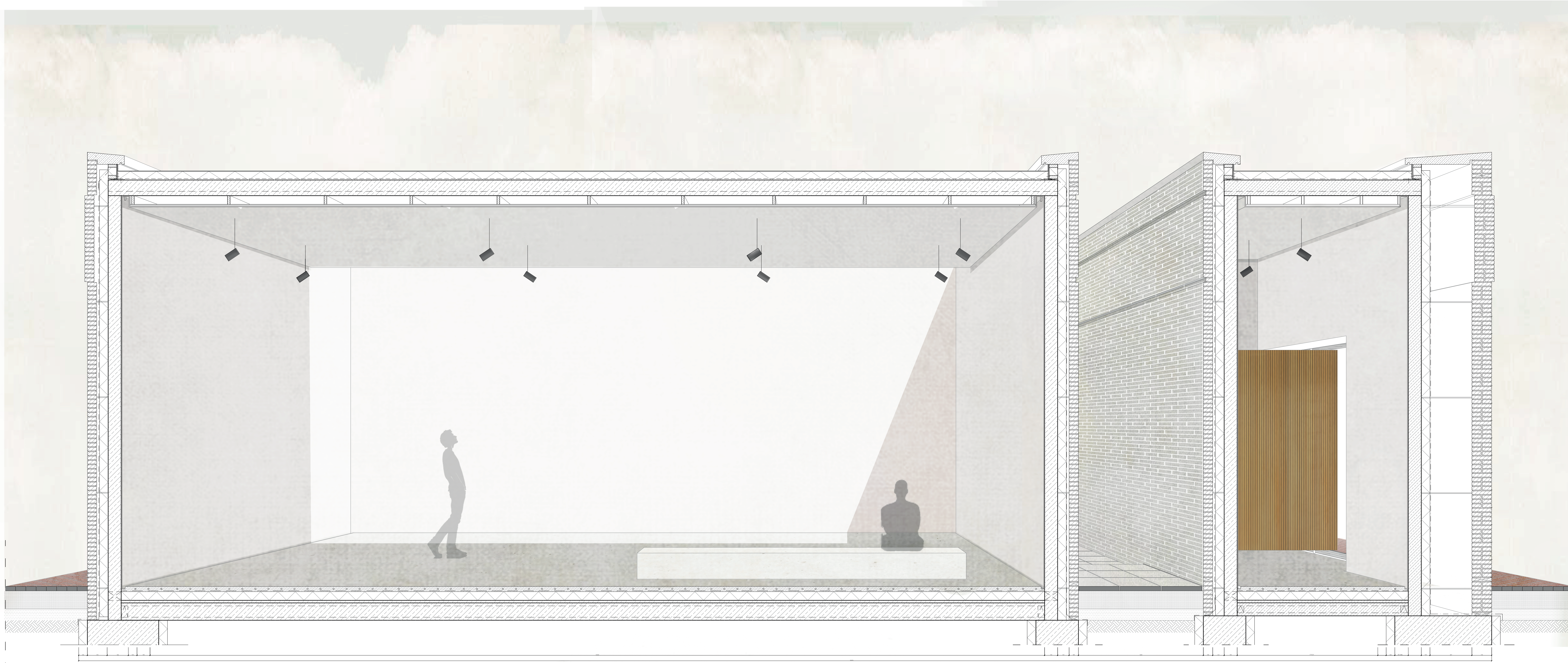
Doorsneden A, 1:20
