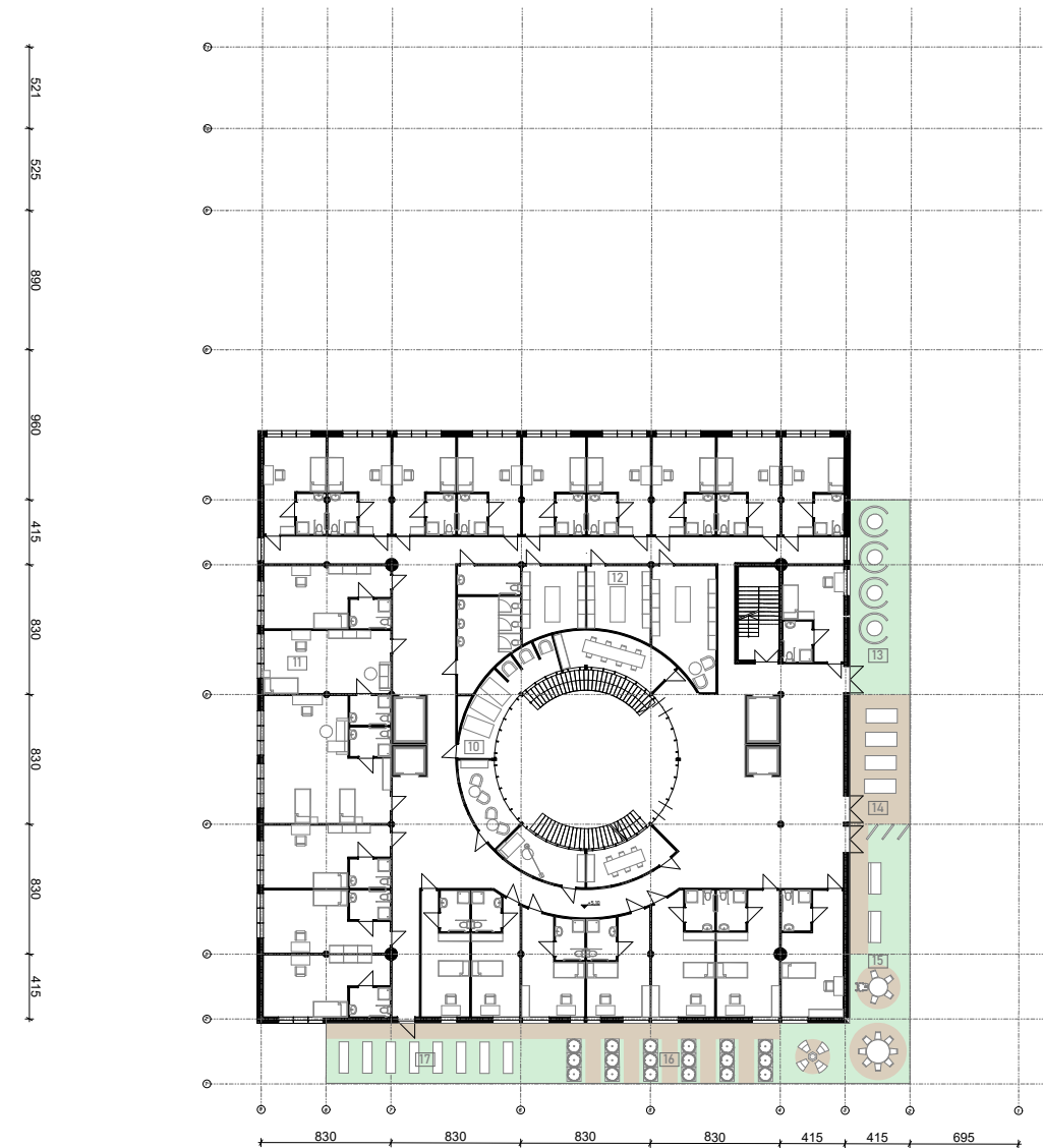
Floor +1 1:200
