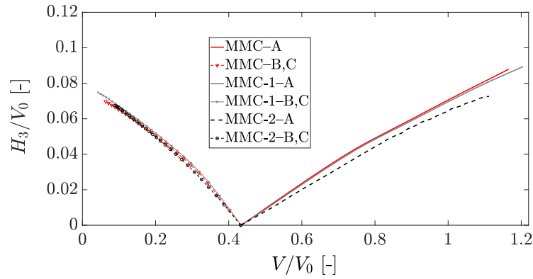
(a) horizontal-vertical ( H_3/V_0 - V/V_0 )
