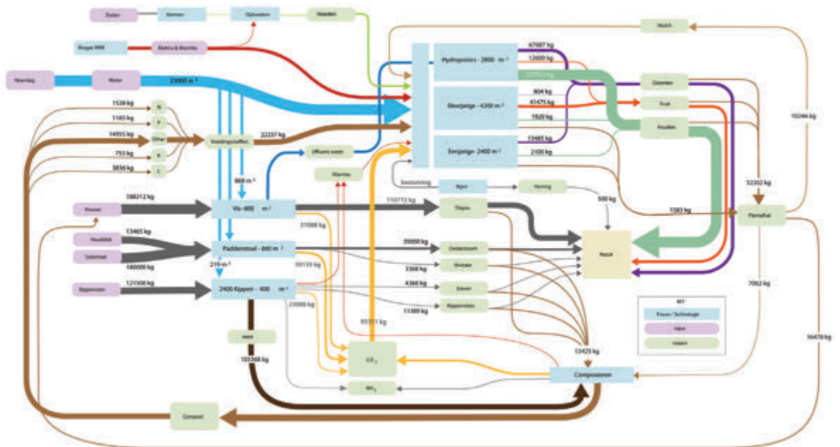
FIG. 4 Materiaalstromen voor een Polydome op 10.000 m² kas. Uit: Polydome 2011, InnovatieNetwerk / SIGN, door Except Integrated Sustainability.
