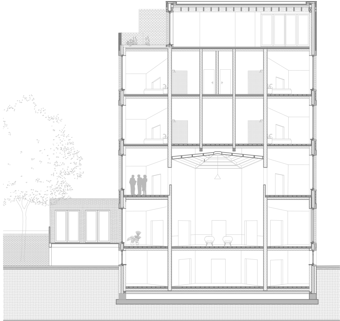
Latitudinal section
