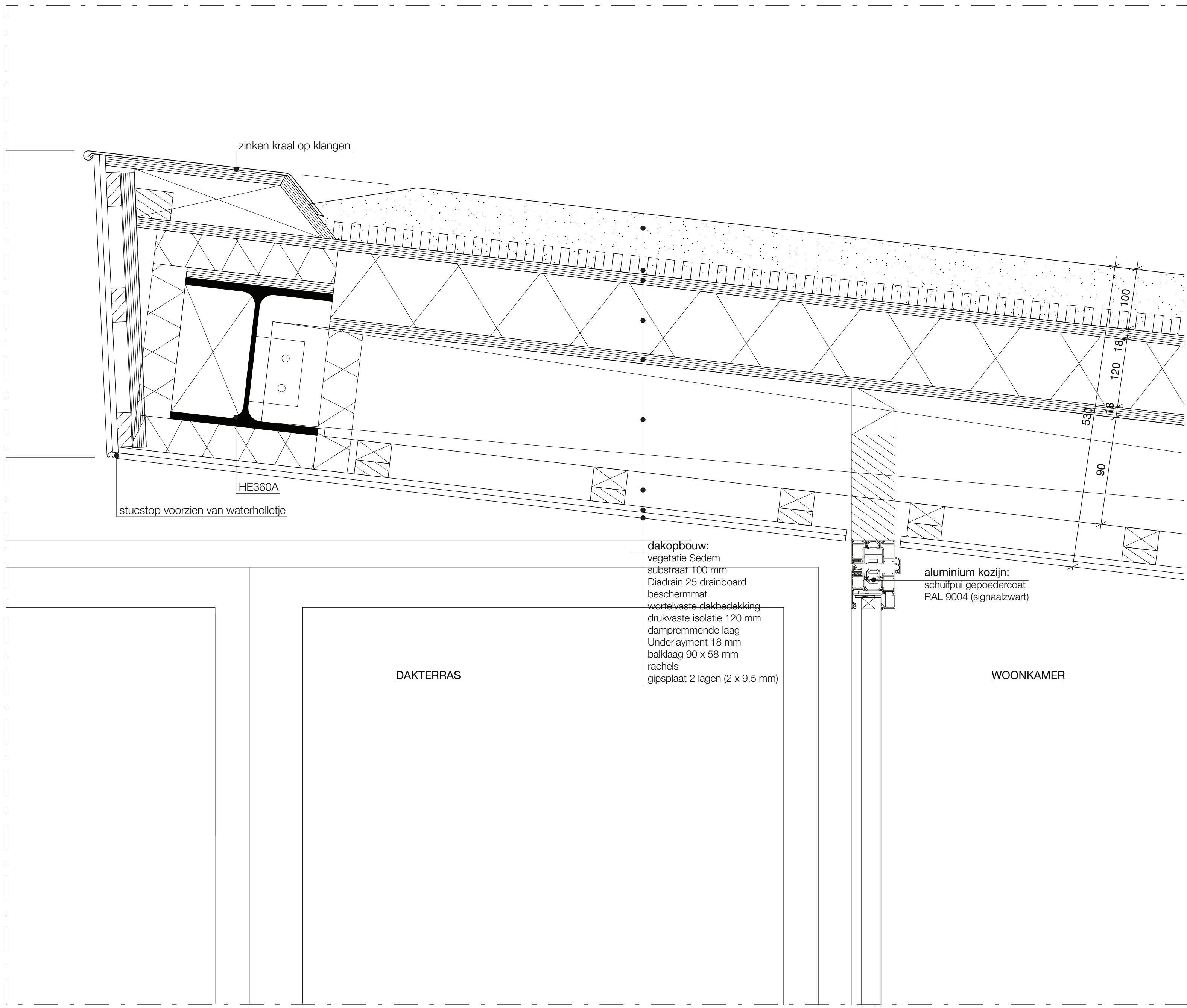
VERTICAAL DETAIL 1 OVERSTEEK DAKRAND 1:5
