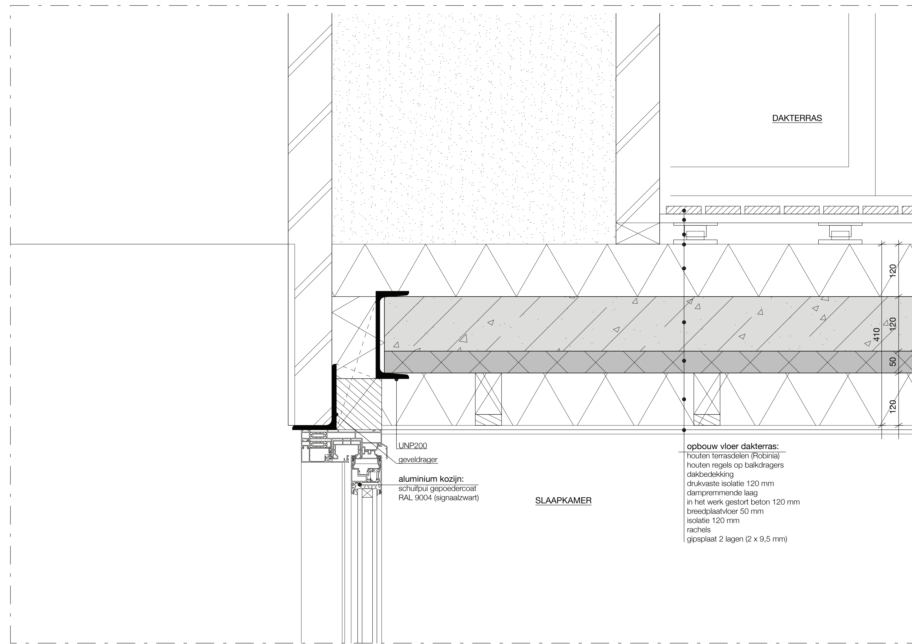
VERTICAAL DETAIL 3 AANSLUITING SCHUIFPUI OP DAKTERRAS 1:5
