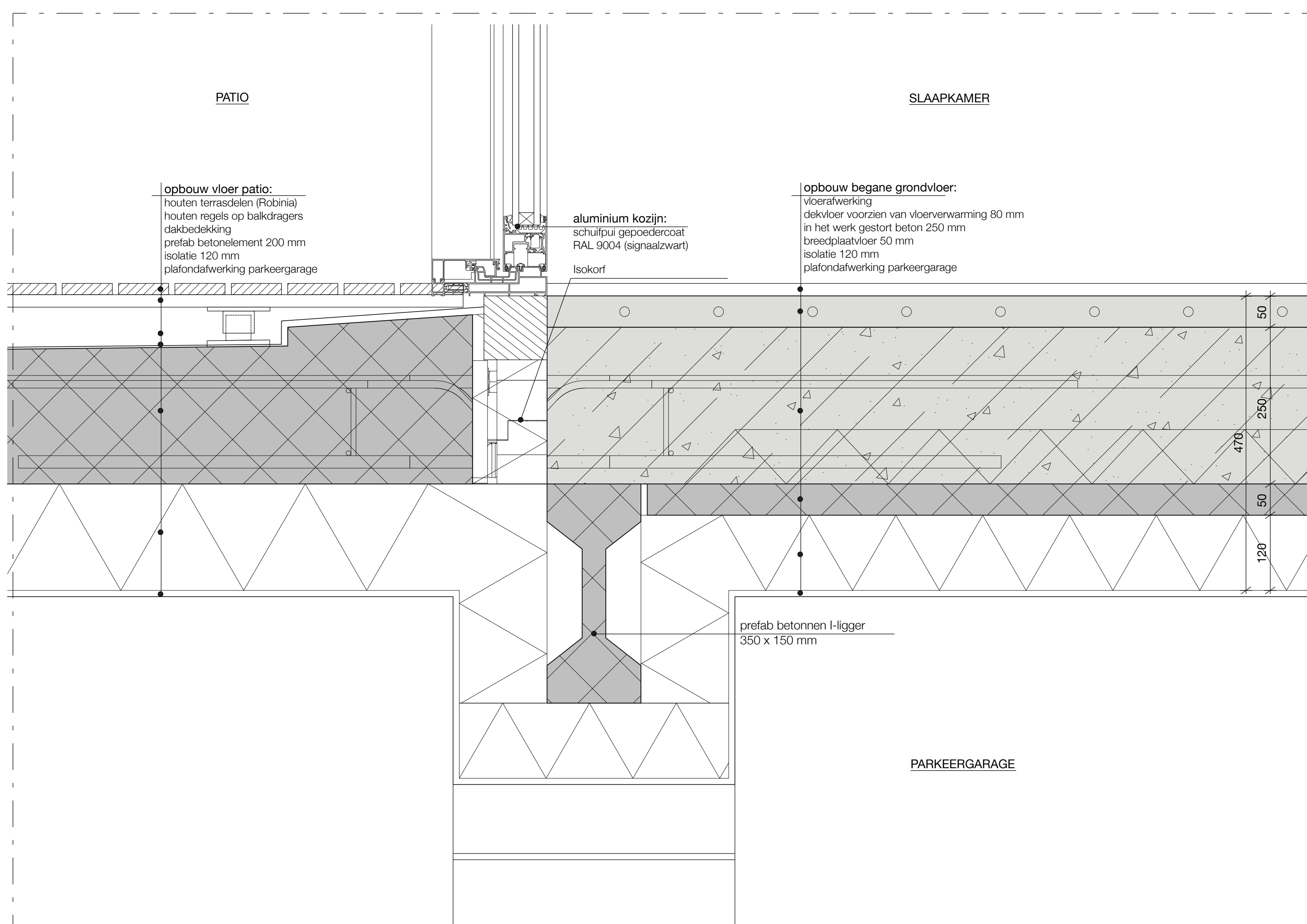
VERTICAAL DETAIL 4 AANSLUITING PATIO OP SLAAPKAMER 1:5
