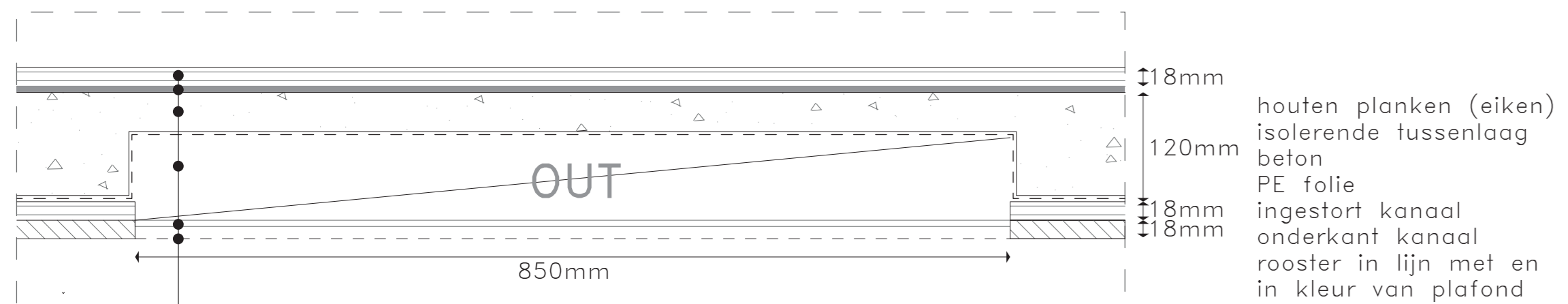
1. ROOFTOP 1:5
