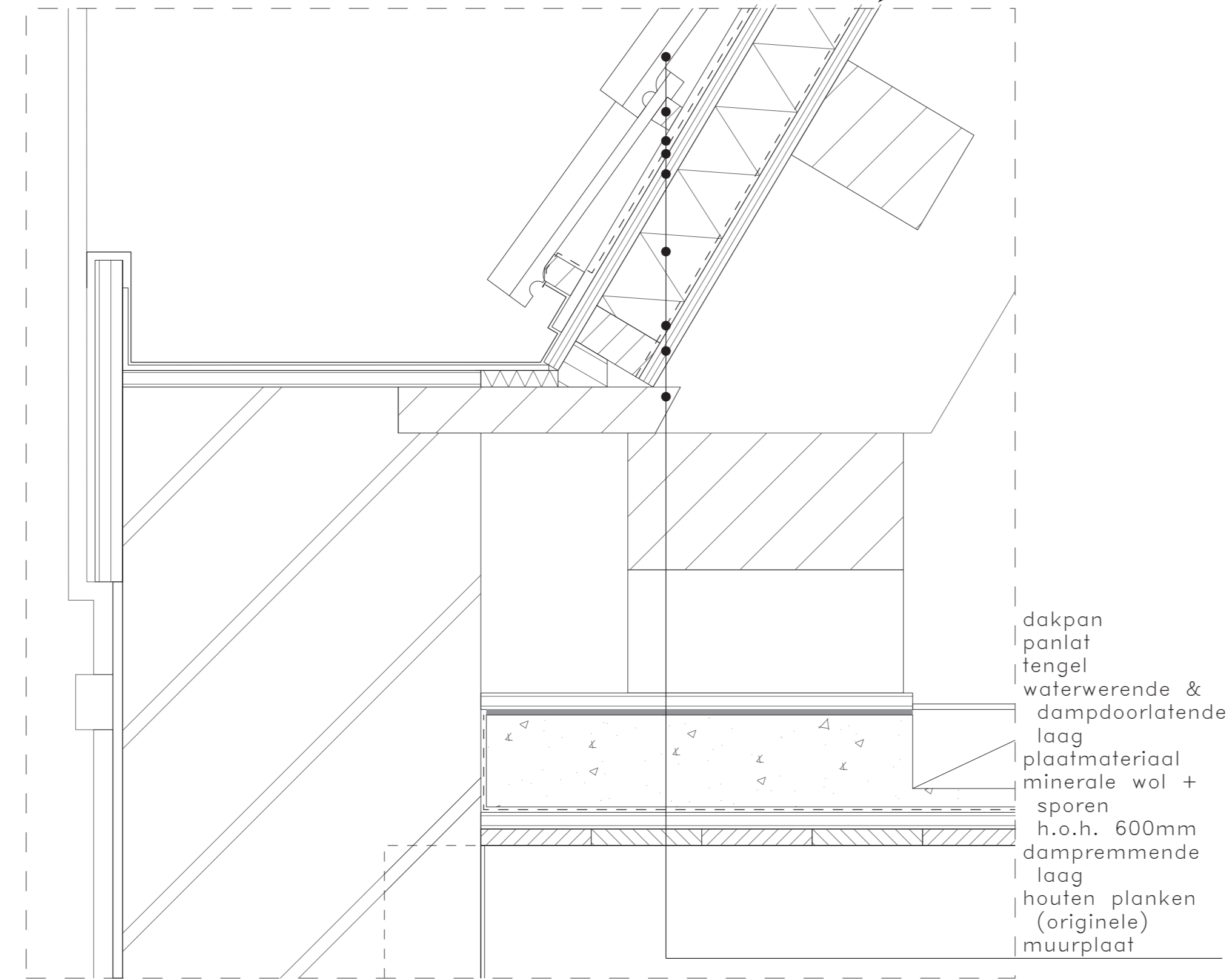
2. ROOF EDGE 1:5
