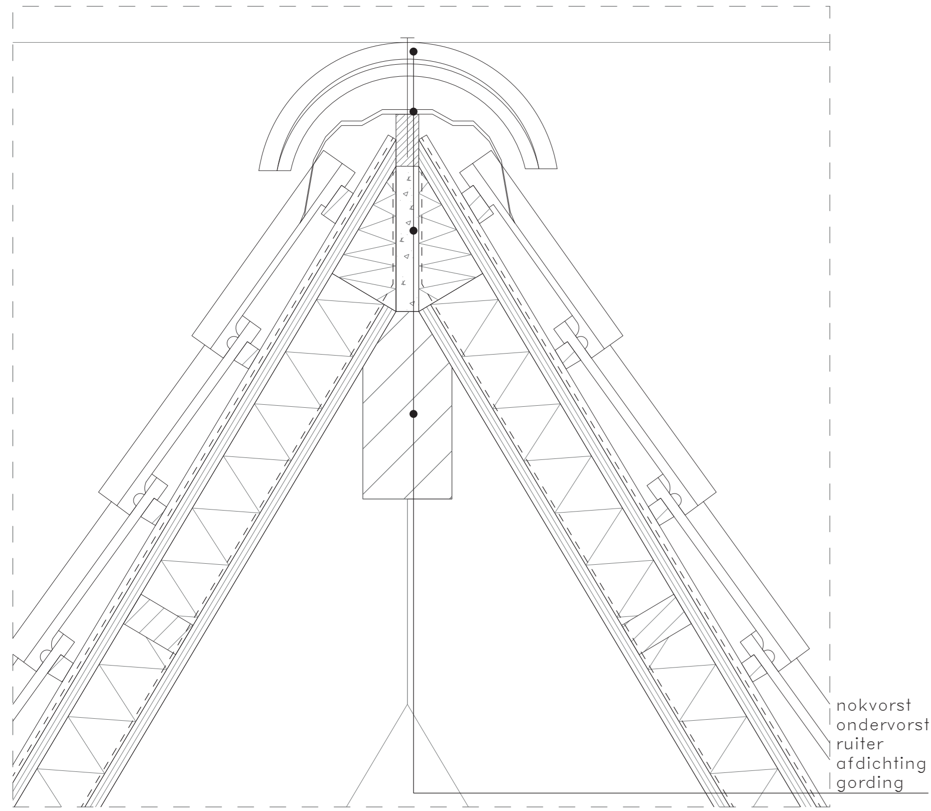
1. ROOFTOP 1:5
