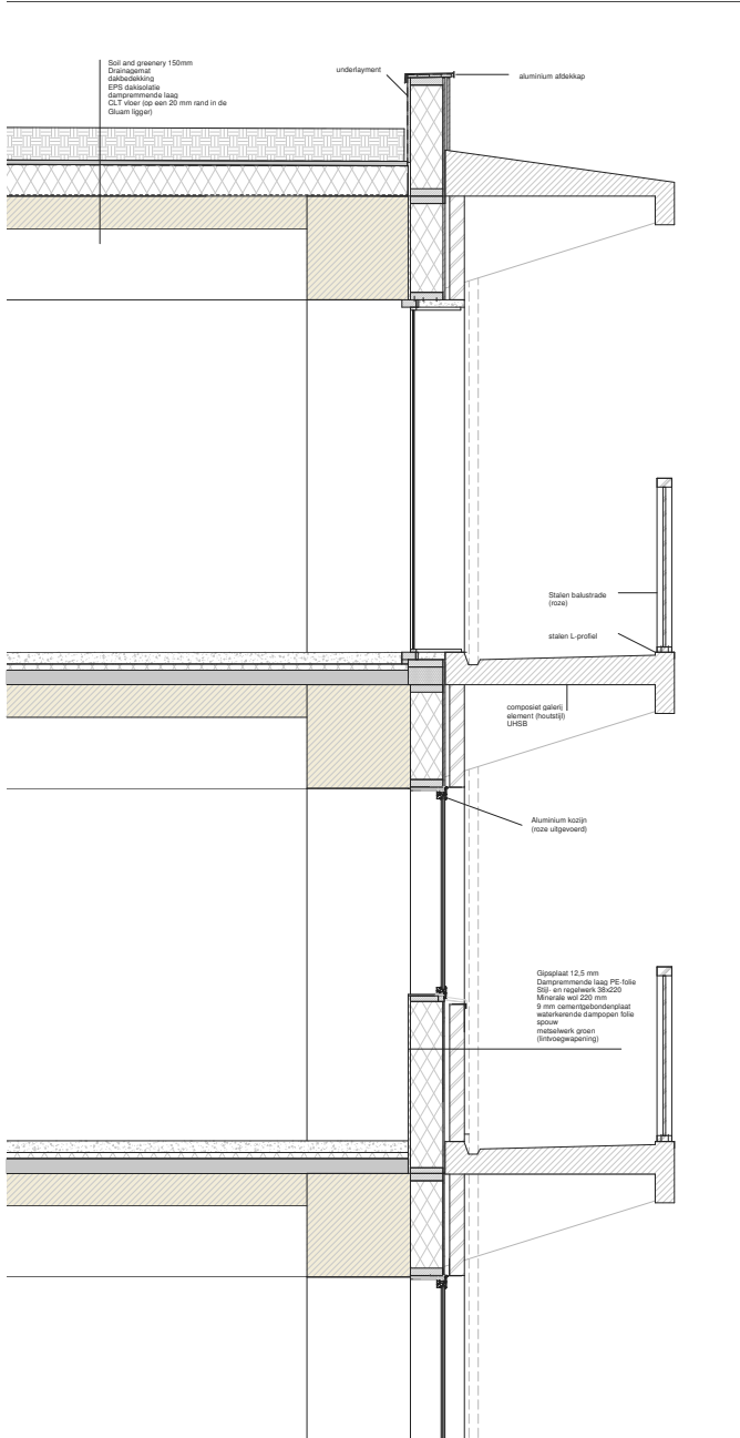
section 1 : 20
