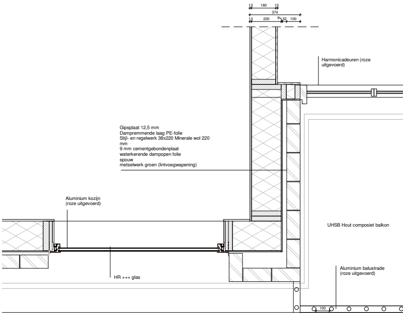
Horizontal detail 1 : 10
