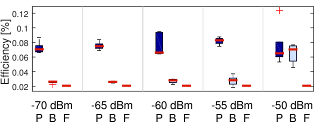
(d) WPTN Efficiency
