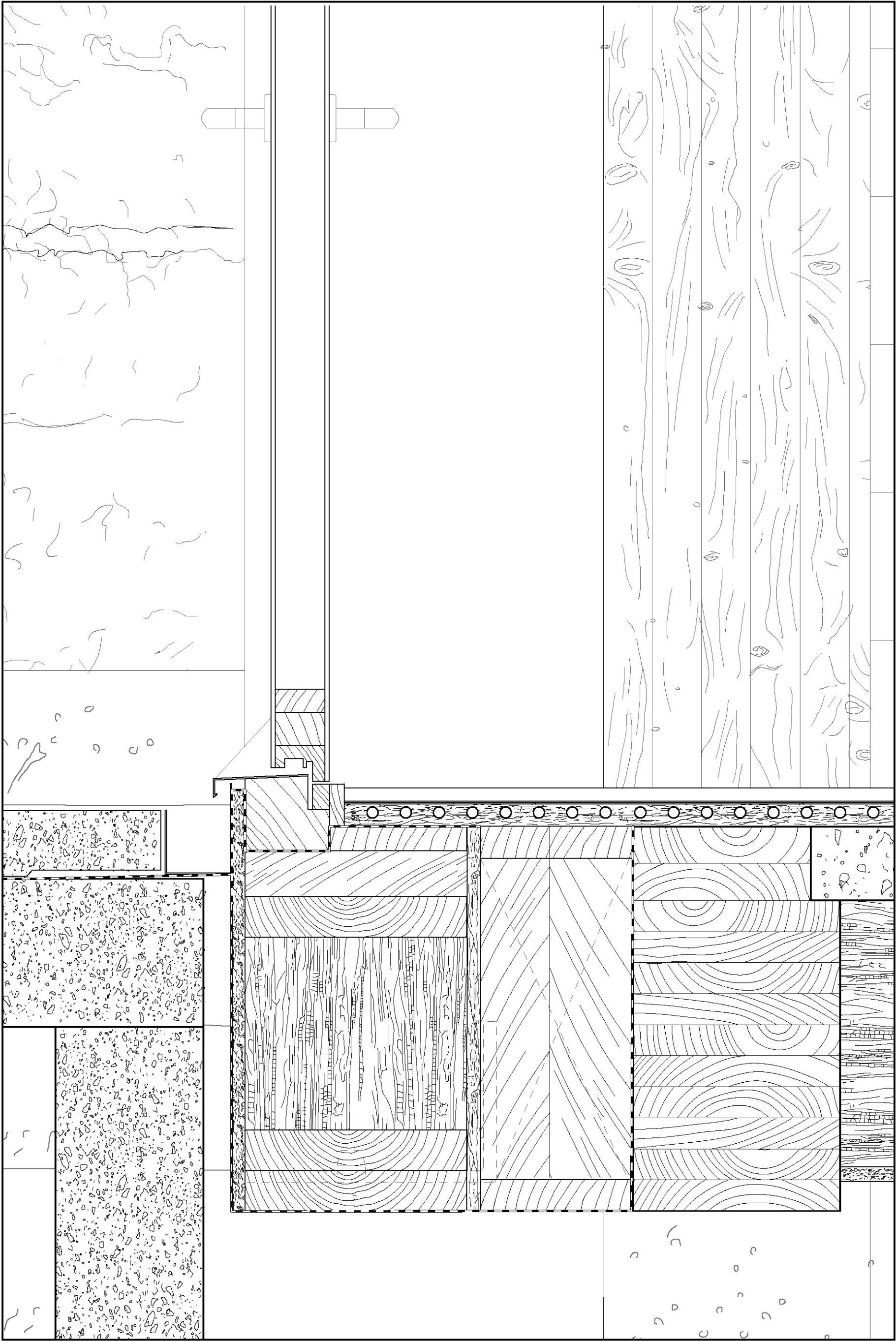
Door Detail 1:5
