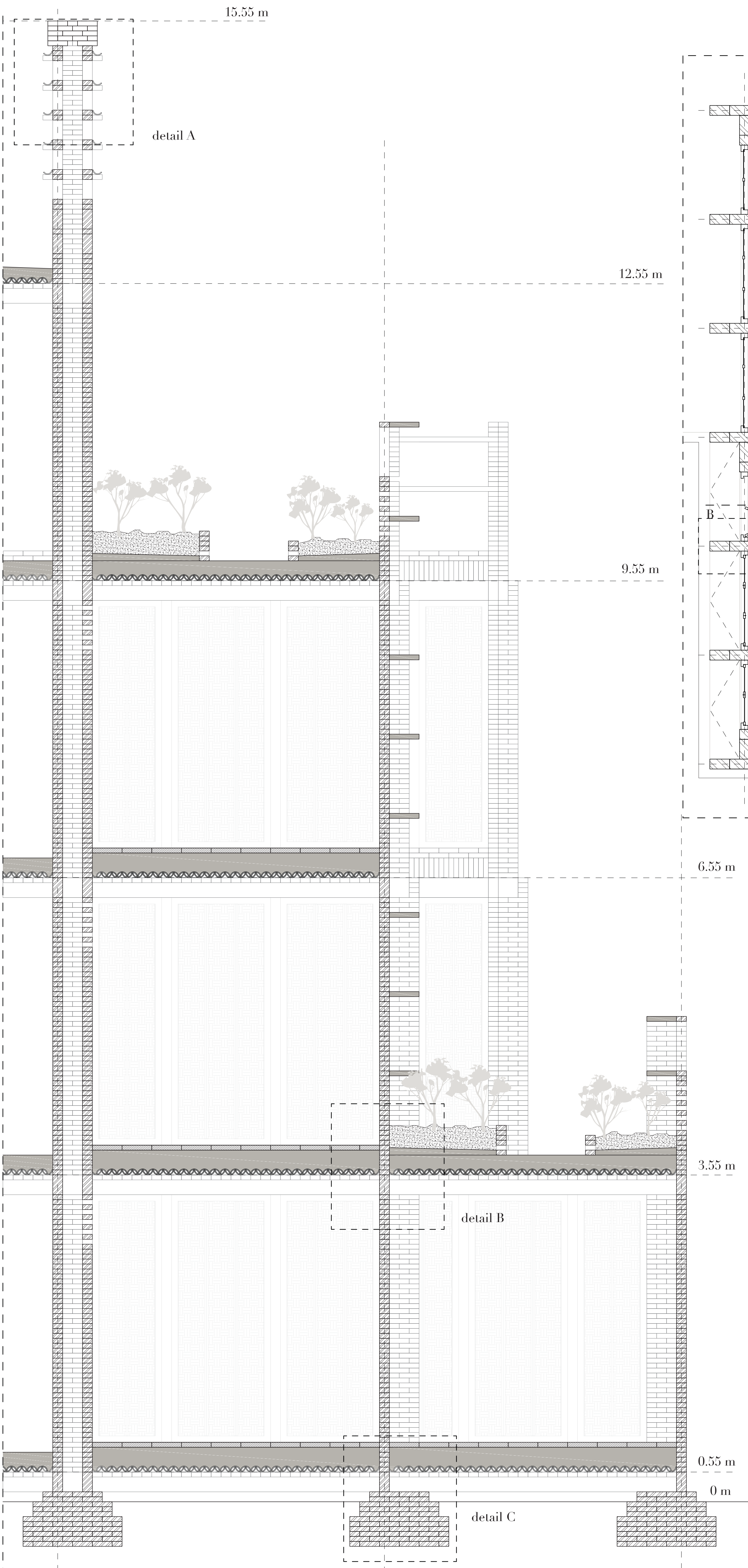
section A-A' 1:20
