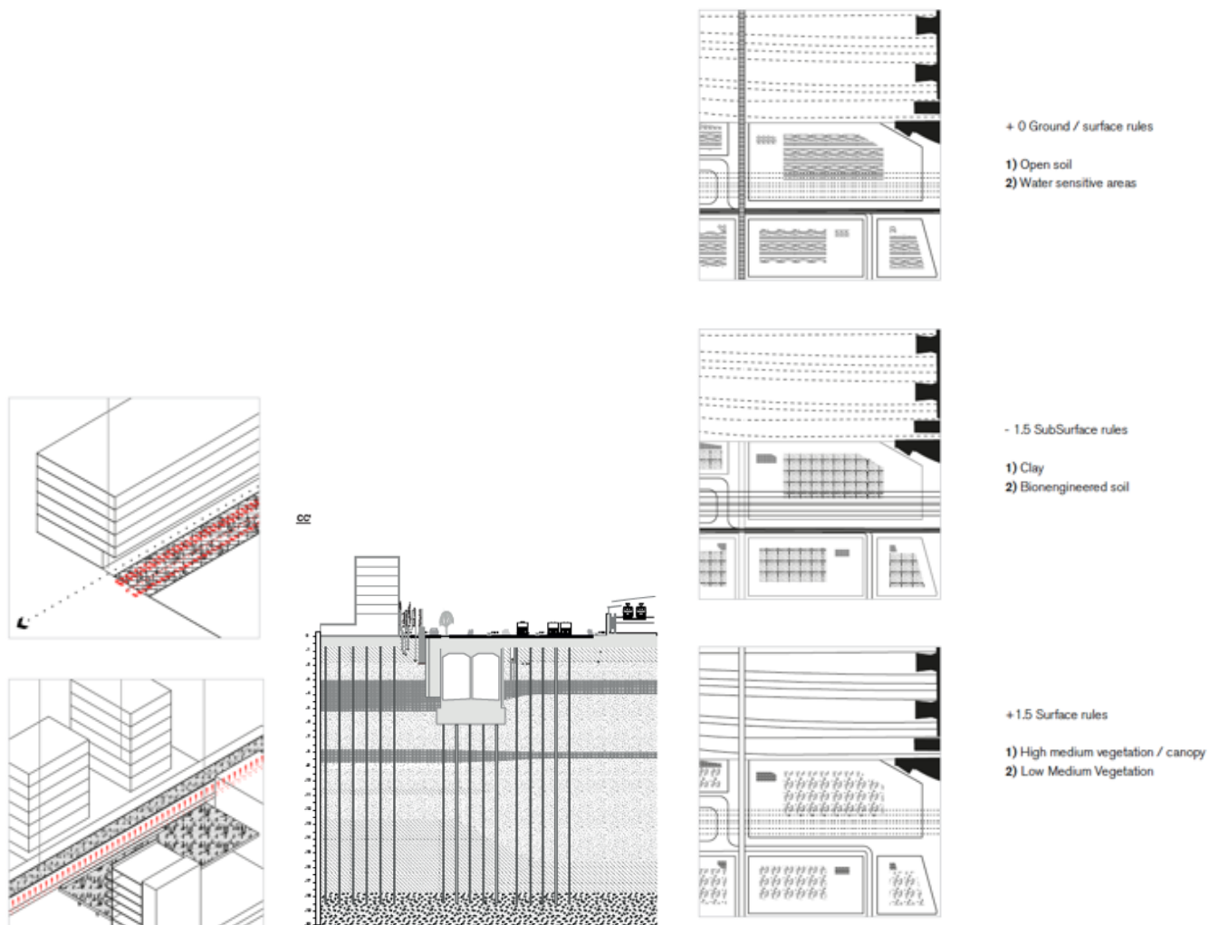
Figuur 31: Relatie tussen axonometrie, doorsnede en verschillende maaivelden in hoog stedelijk gebied (Hooimeijer en Lafleur, 2018b)
