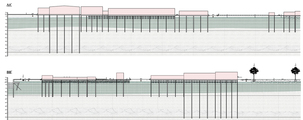
Figuur 36: Technisch profiel casus Oostende (een leesbare versie is opgenomen in appendix 6)
