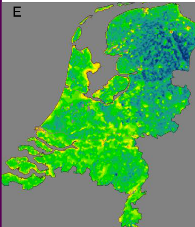
De ongebruikelijke methode van TNO om hitte-eilanden te bepalen: C. Nachtelijk NOAA satellietbeeld. D. Verwijderen stedelijke pixels (1km x 1km), E. Opvullen van de lege delen door middel van interpolatie. F. Kaart E in mindering gebracht op kaart C.
