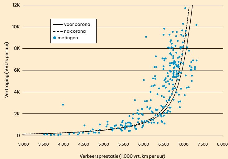
Figuur 12: Idem als in figuur 11, maar nu met de geschatte relaties tussen verkeersprestatie en vertraging ingetekend (bron: Rijkswaterstaat).
