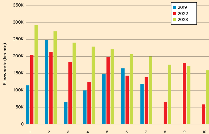
Figuur 4: De filewaarde van de grootste knelpunten van 2023 (File Top 10) voor respectievelijk 2019, 2022 en 2023.
