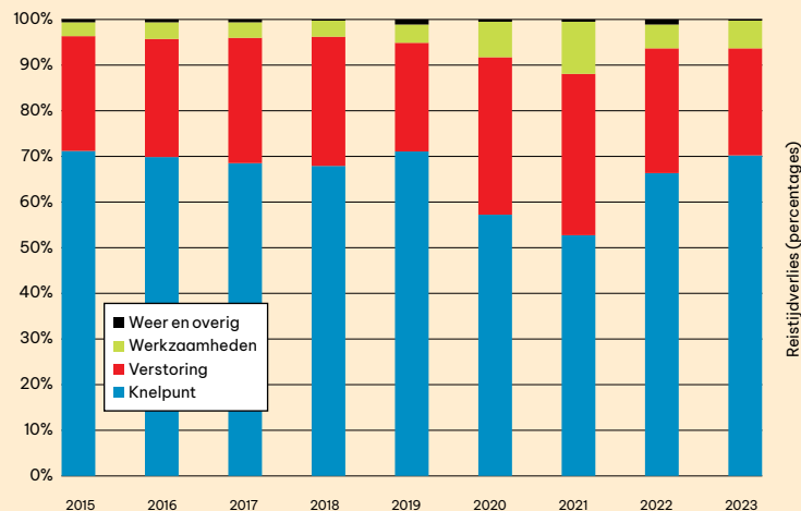
Figuur 3: Reistijdverlies naar oorzaak, relatief (bron: Rijkswaterstaat).
