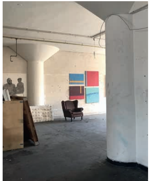
16. J.E. Ferguson en S. Stakesby-Lewis, interieur van het voormalige kantoorgebouw August House in Doornfontein, Johannesburg, in 1946 ontworpen en nu kunstenaarshuis. Imposante draagconstructie van ronde paddenstoelkolommen met conische koppen (collectie August House, Johannesburg)
