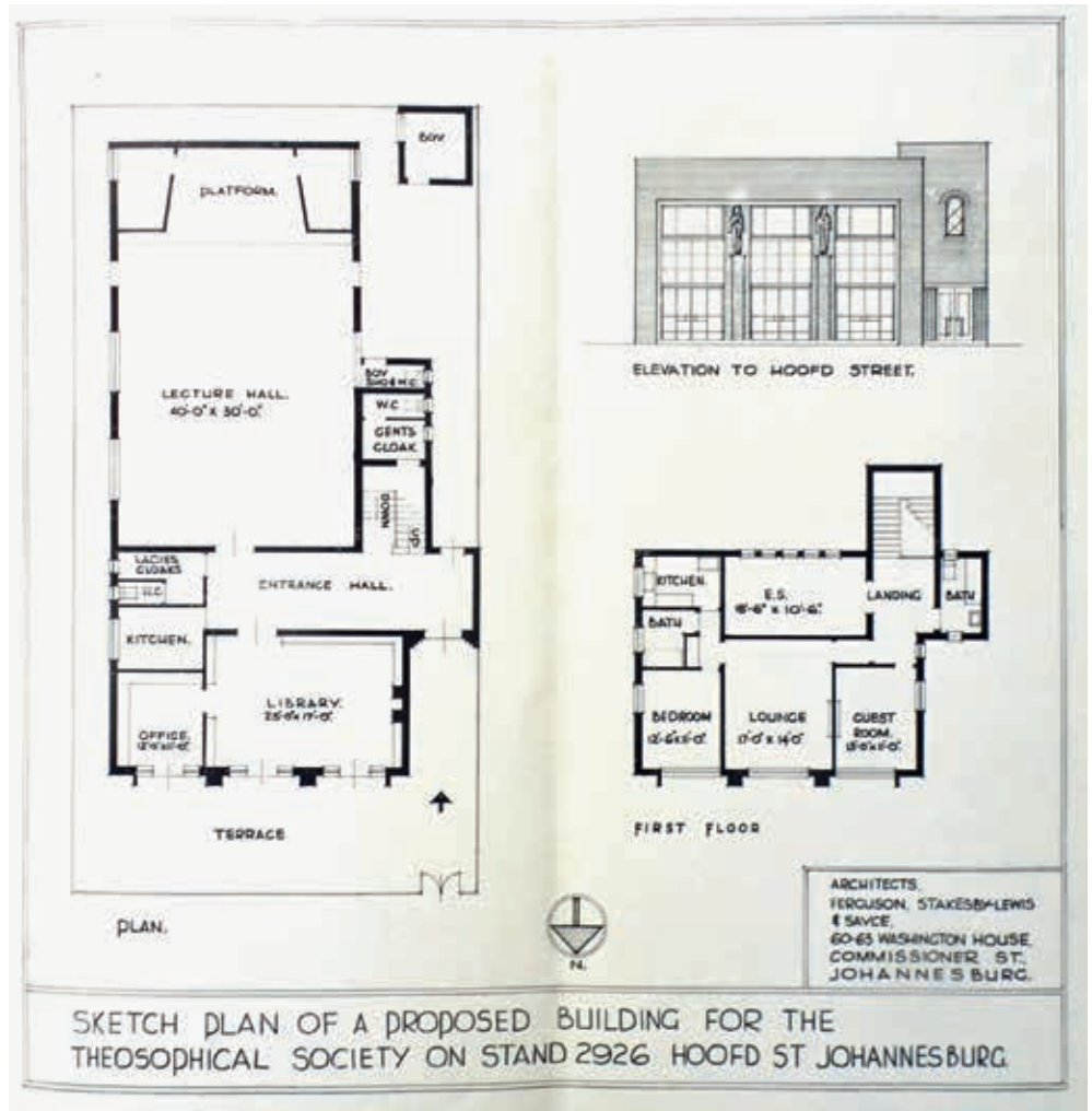
19. Ferguson, Stakesby-Lewis & Sayce, niet uitgevoerd ontwerp voor een nieuw logegebouw voor de Theosophical Society aan de Hoofdstraat in Johannesburg, 1949 (jubileumboek Fifty Years of Theosophy , 1949)
