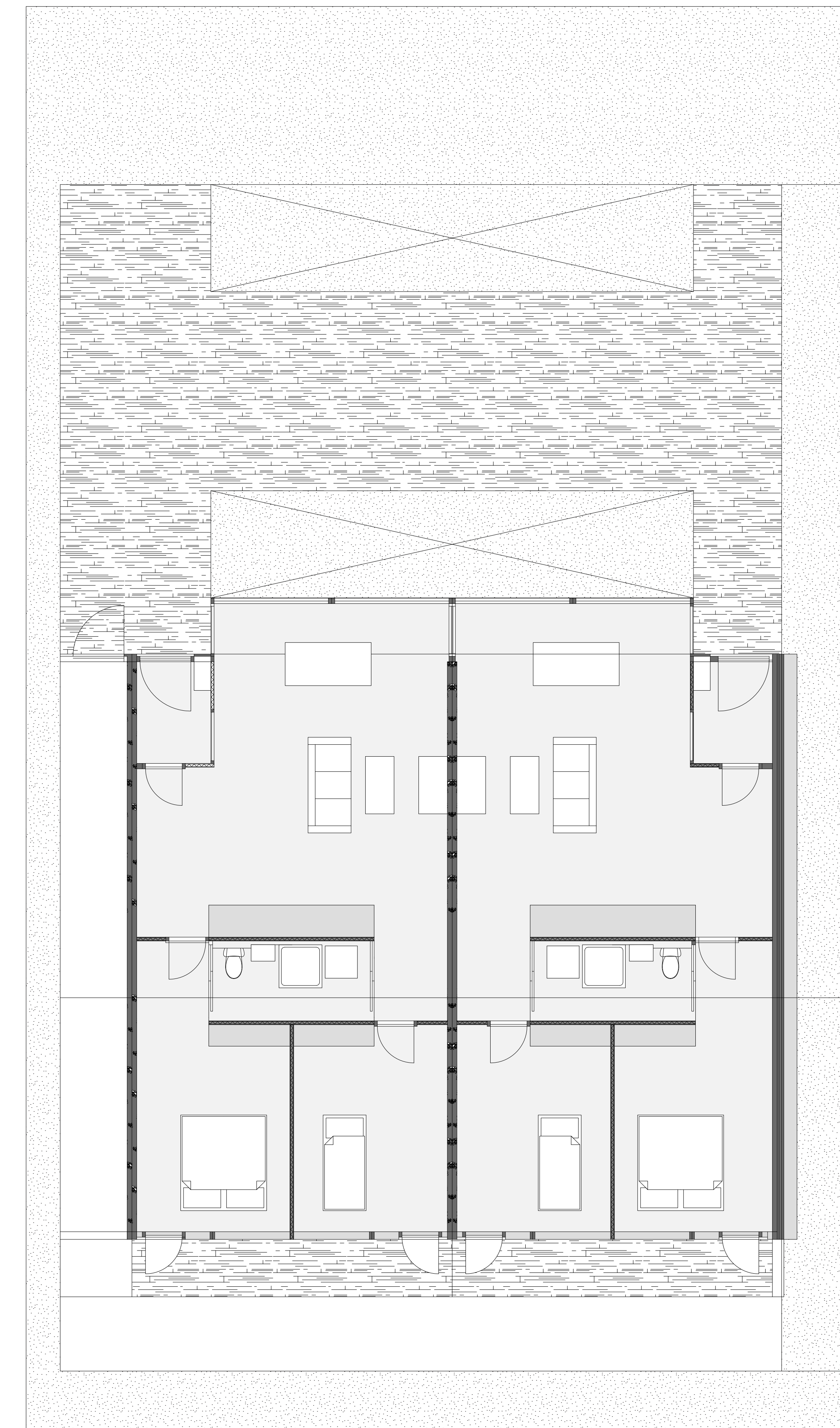
Plattegrond energievlugel 1:50
