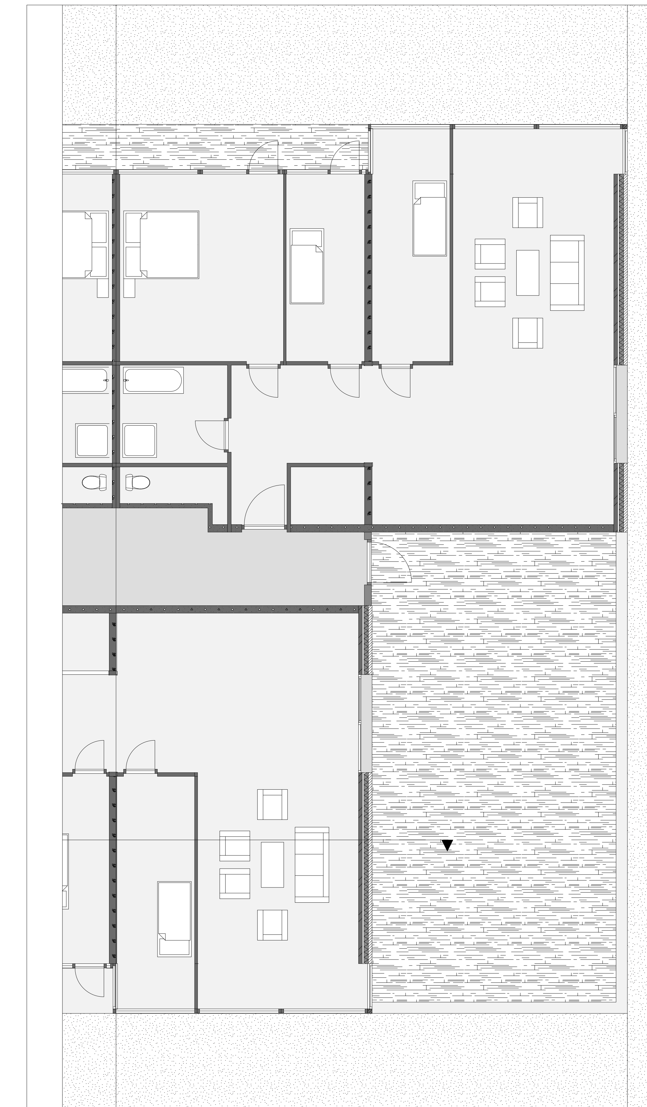
Plattegrond appartementenvleugel 1:50
