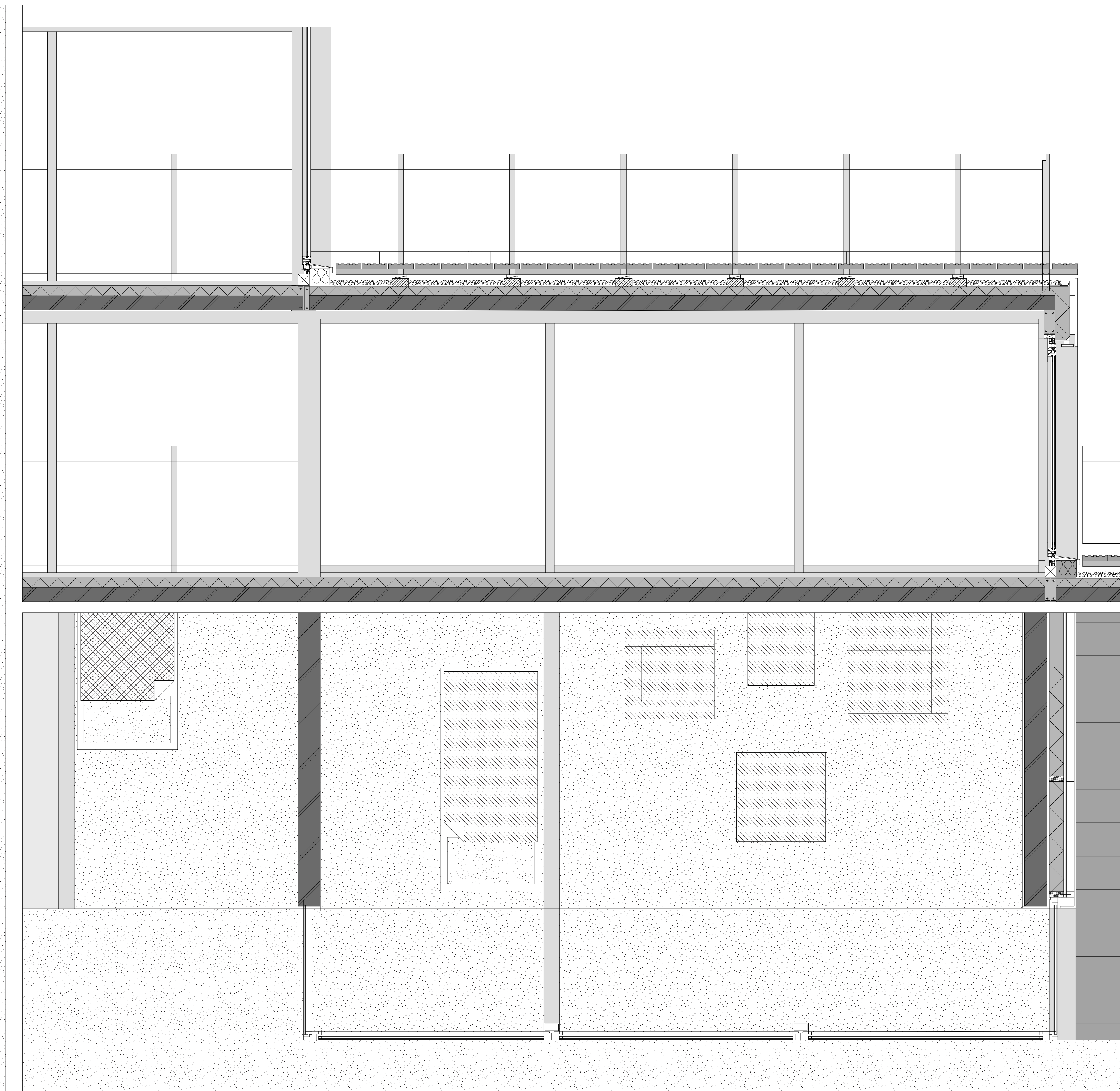
Doorsede 1:20 appartementen vleugel
