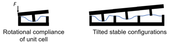
(d) 3D unit cell – rotational compliance
