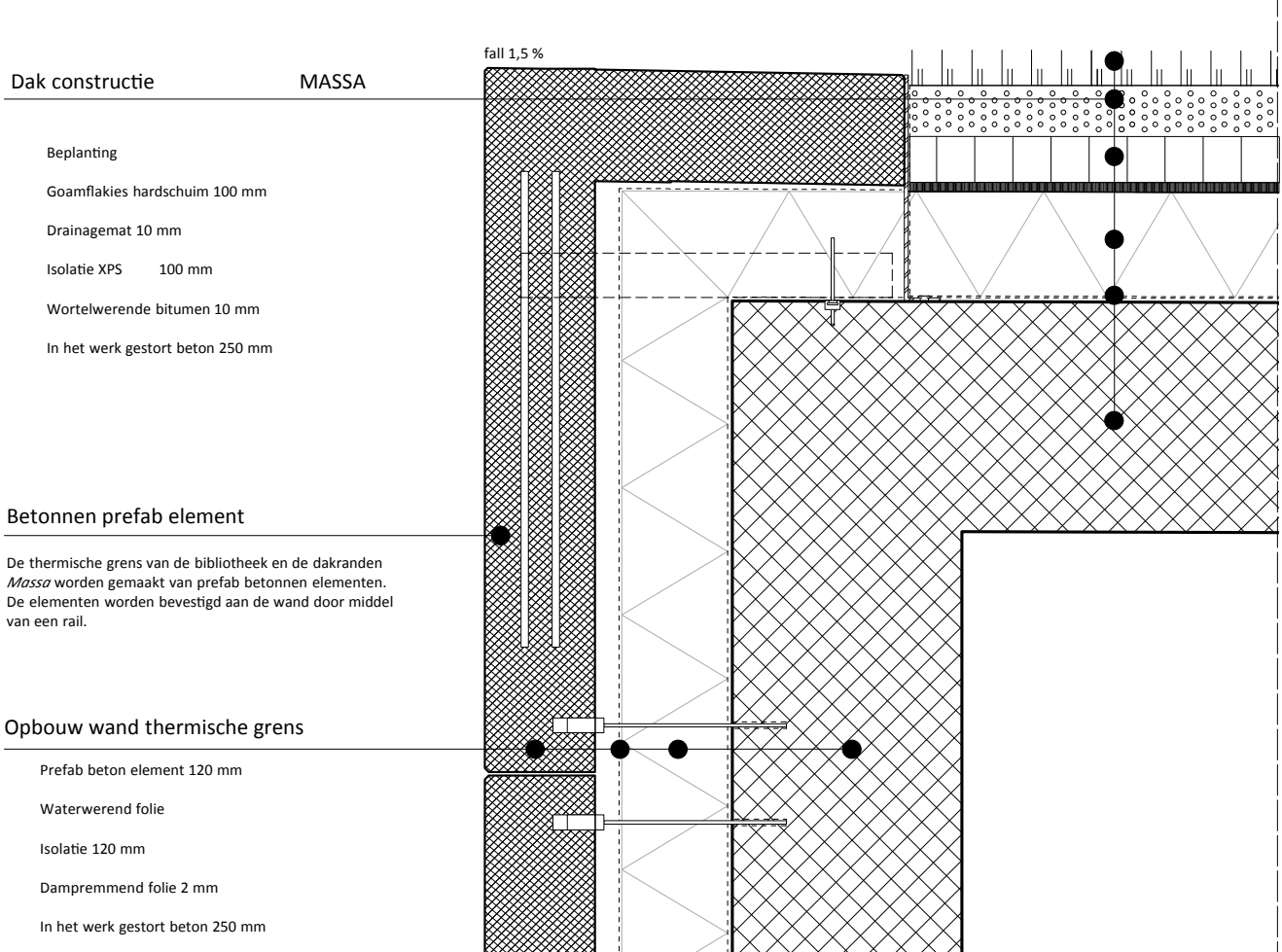
Detail V1 Dakrand Massa Wanddikte:
