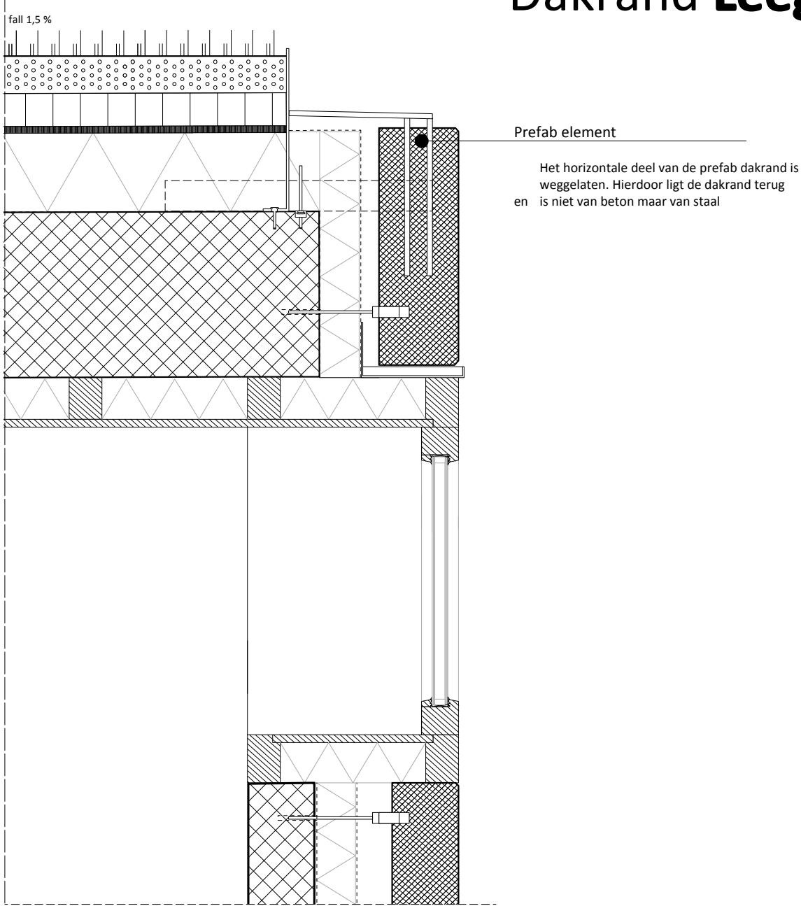
Detail V3 Dakrand Leegte
