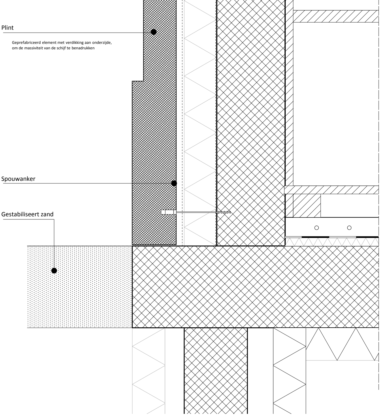
Detail V2 Plint Massa
