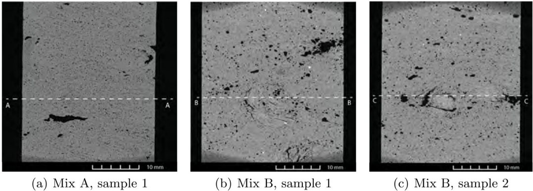
Fig. 16. CT scan images.
