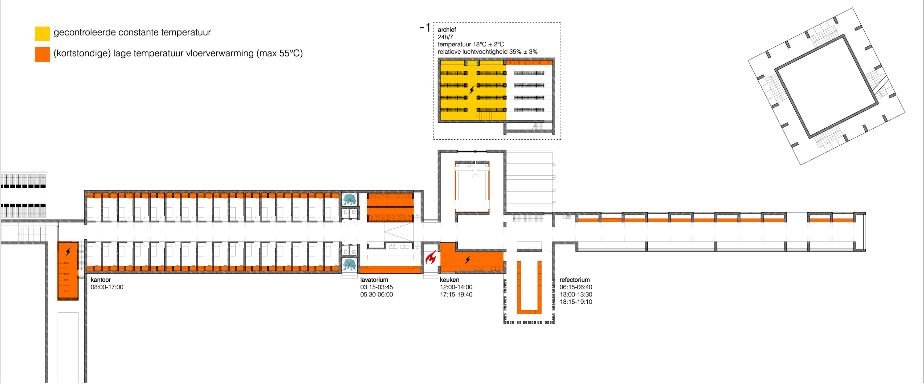
SCHEMA KLIMAAT
