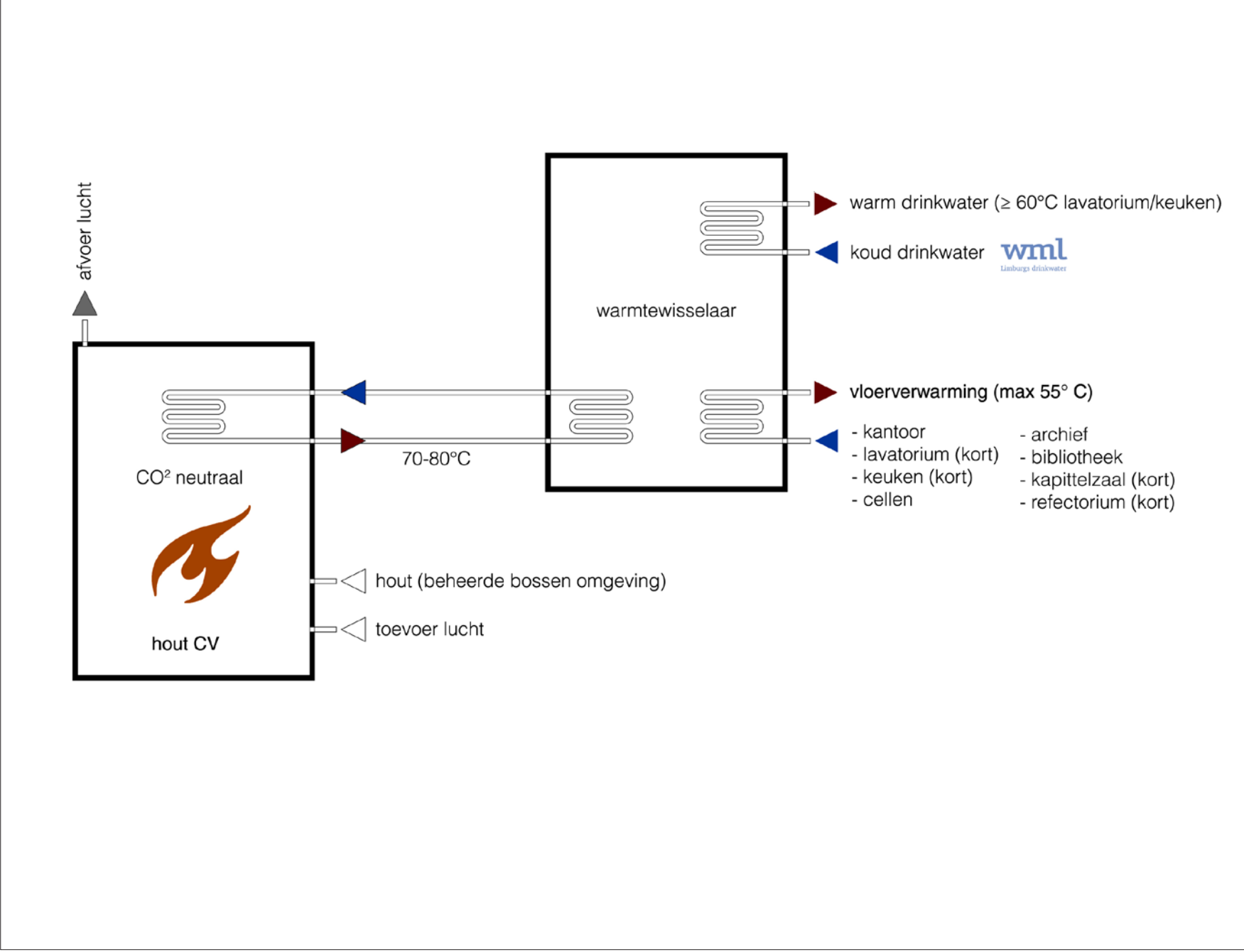
SCHEMA WARMTE
