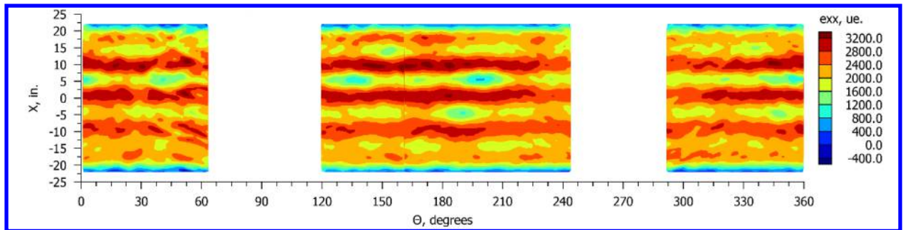
c.) Hoop strain.
