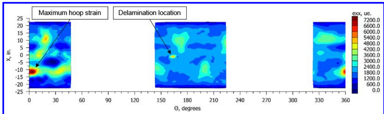
c.) Hoop strain.
