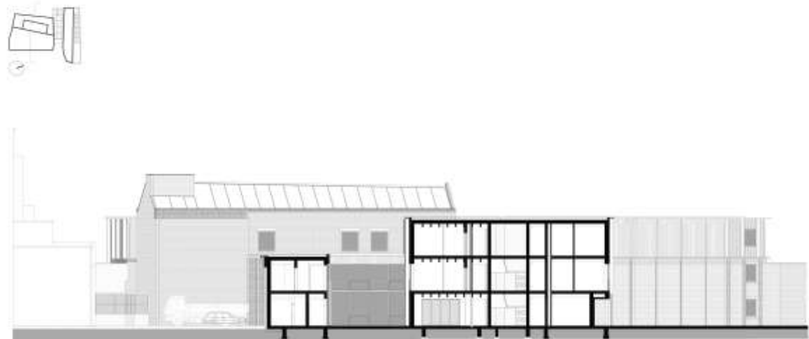
Longitudinal section
