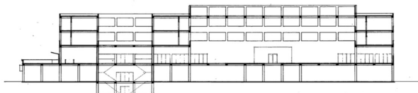
Dwarsdoorsnede
