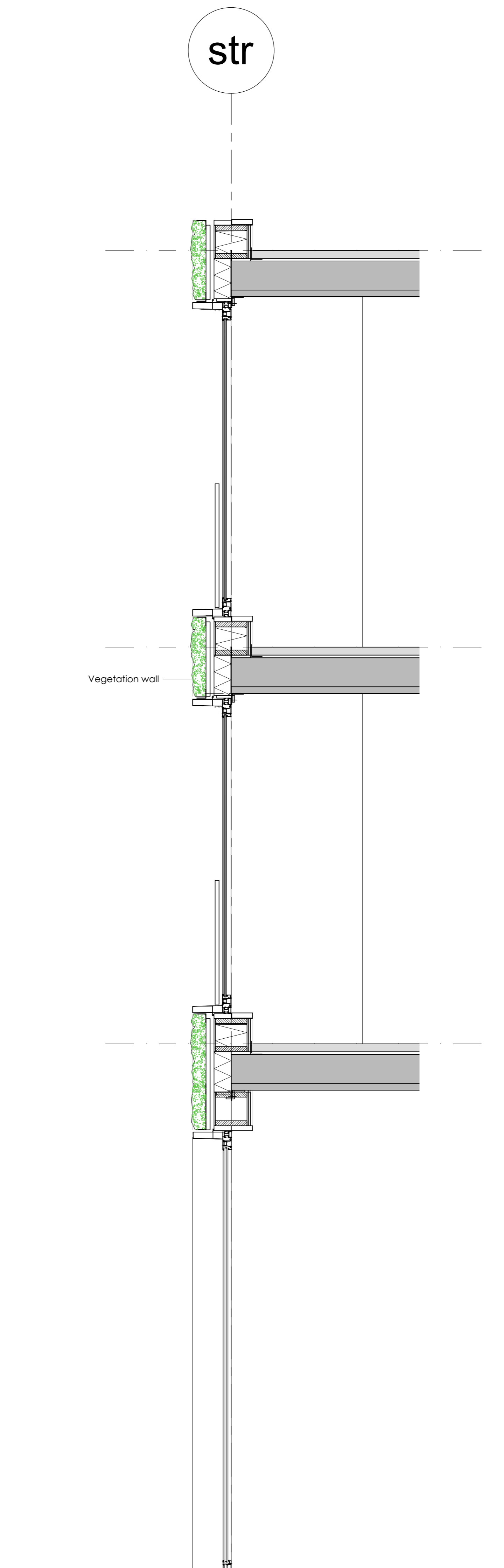
Wall Section A 1 : 20
