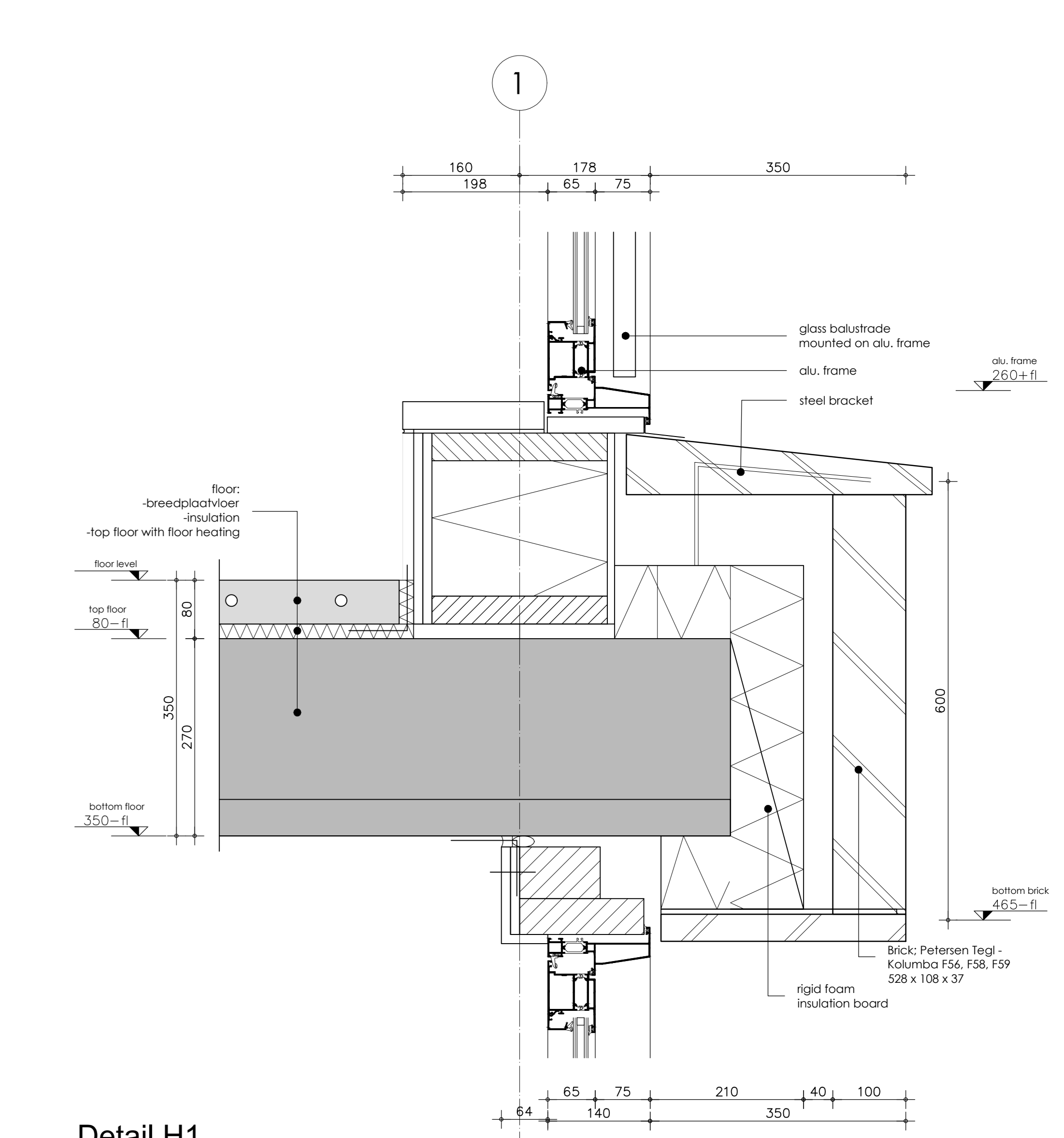
Detail H1 1 : 5
