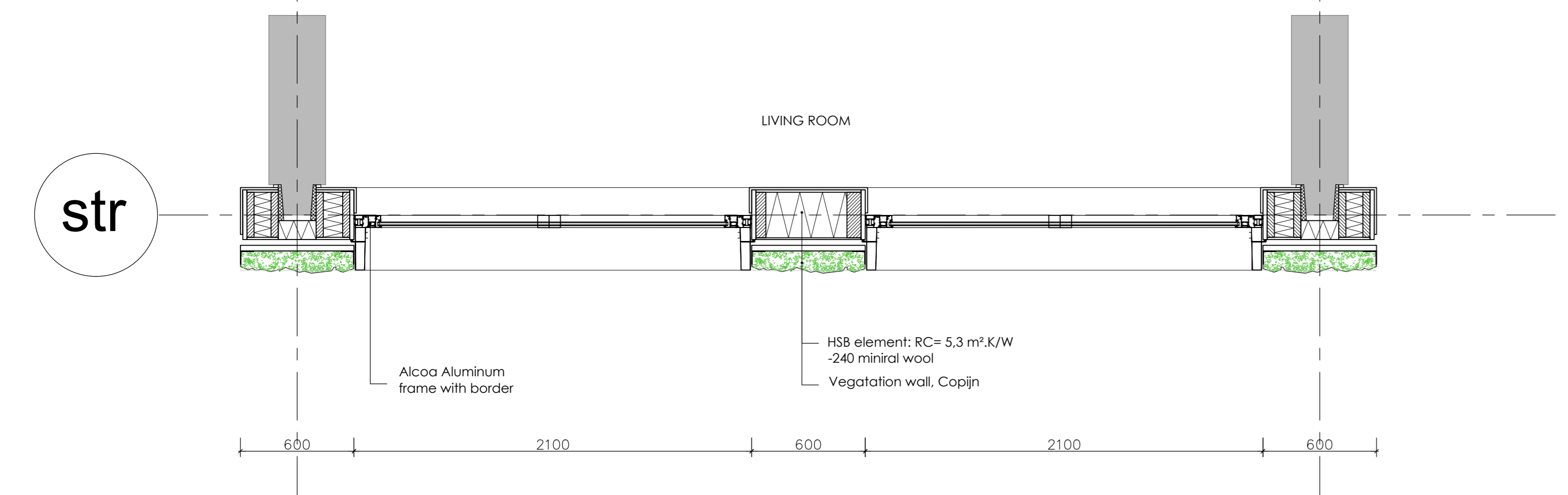
hor. frag 1 : 20
