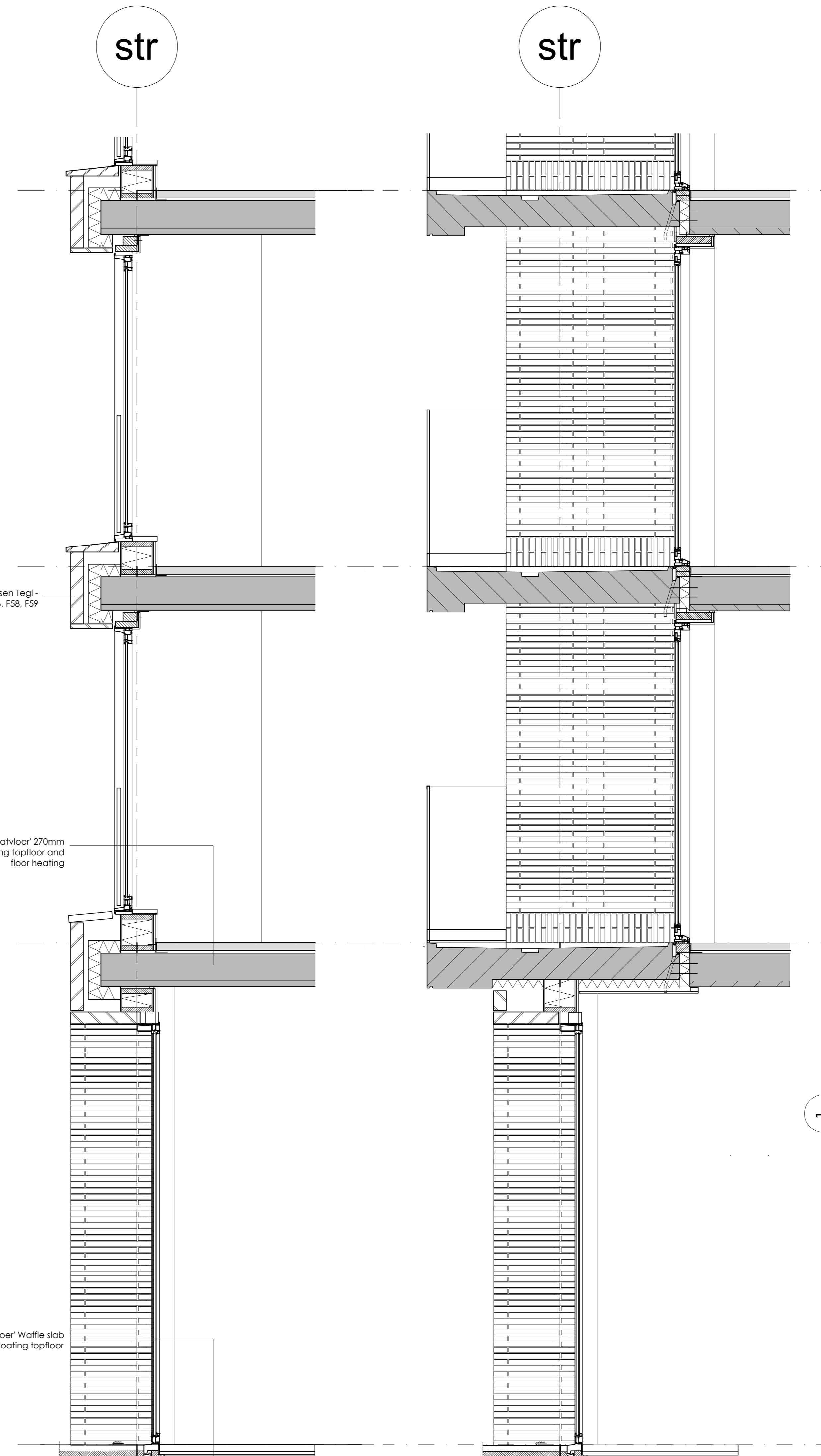
Wall Section A 1 : 20
