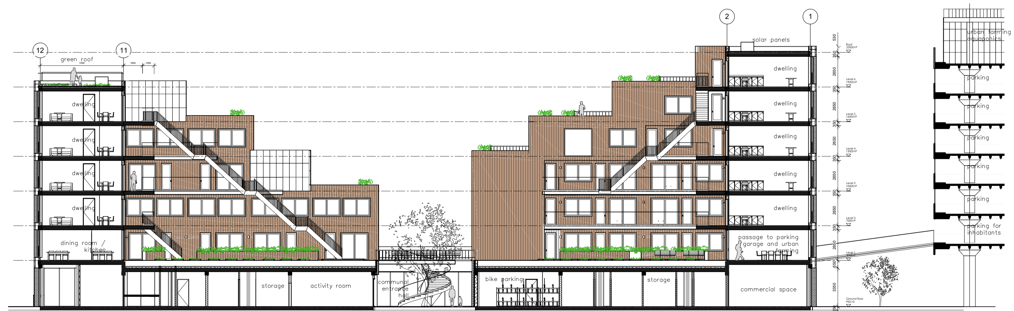
Section DD
