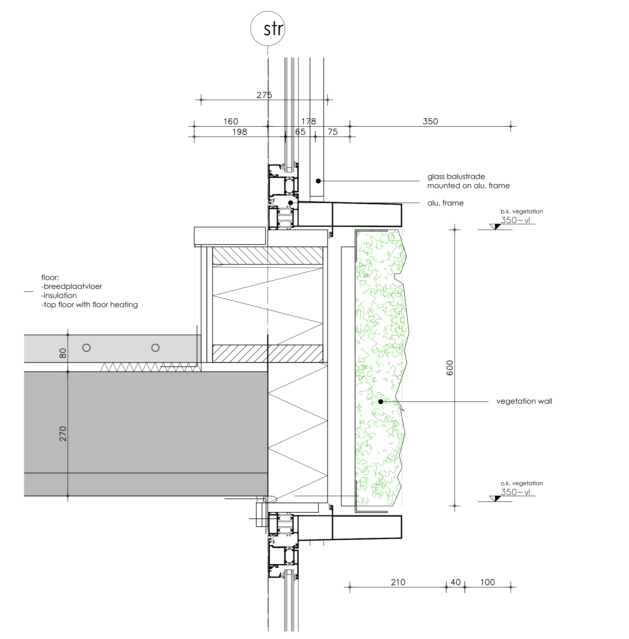
Detail V1 1 : 5
