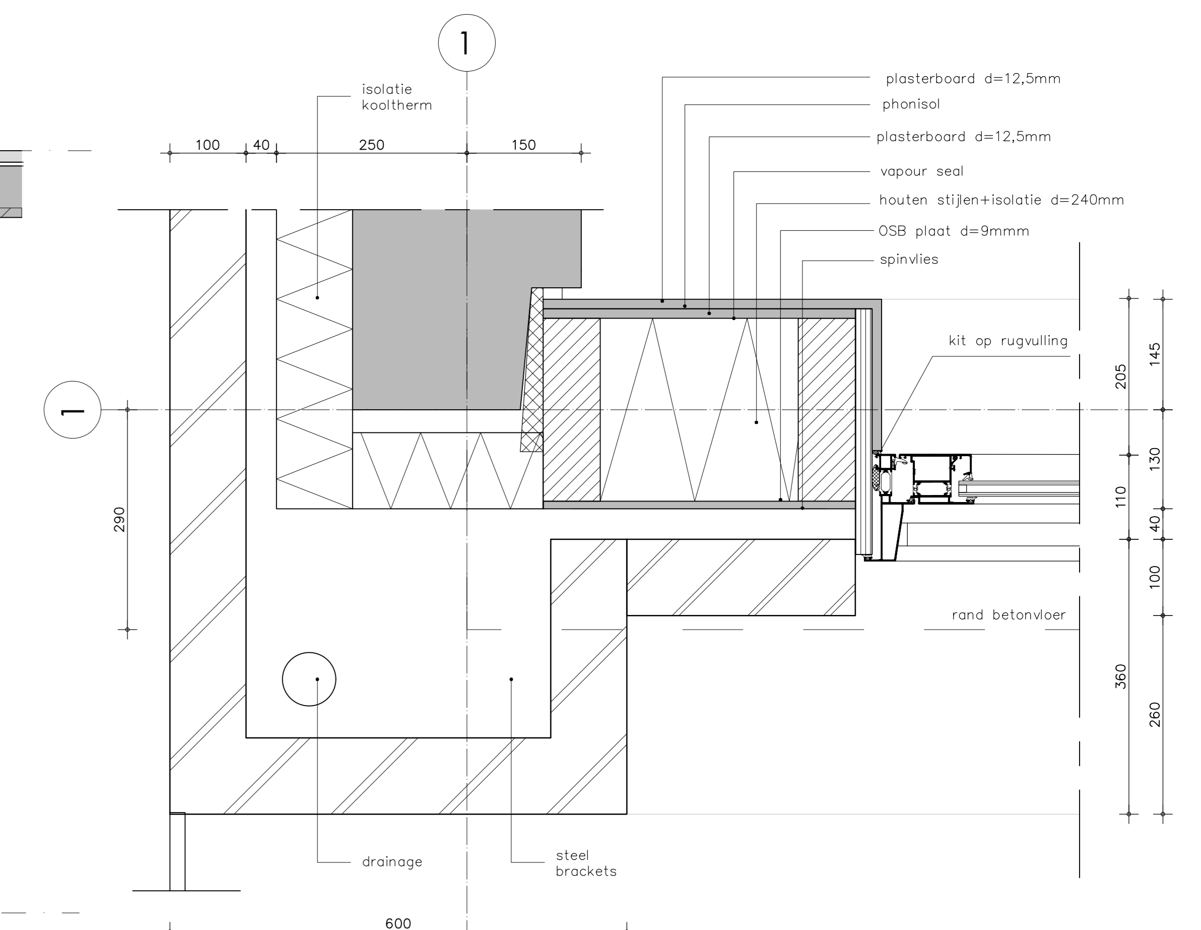
Detail V1 1 : 5
