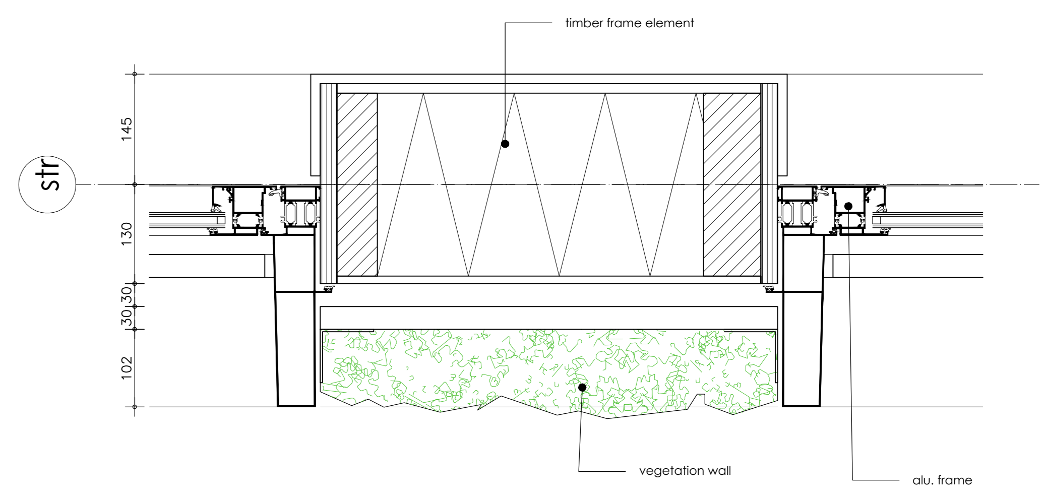
Detail H1 1 : 5
