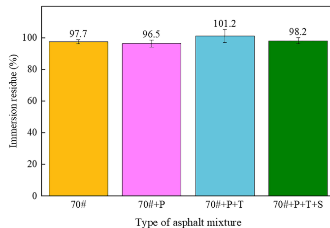
Fig. 13. Immersion Marshall test data.
