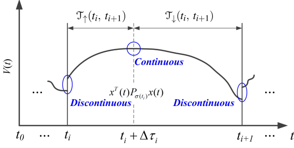
Fig. 1. The Lyapunov function (5).
