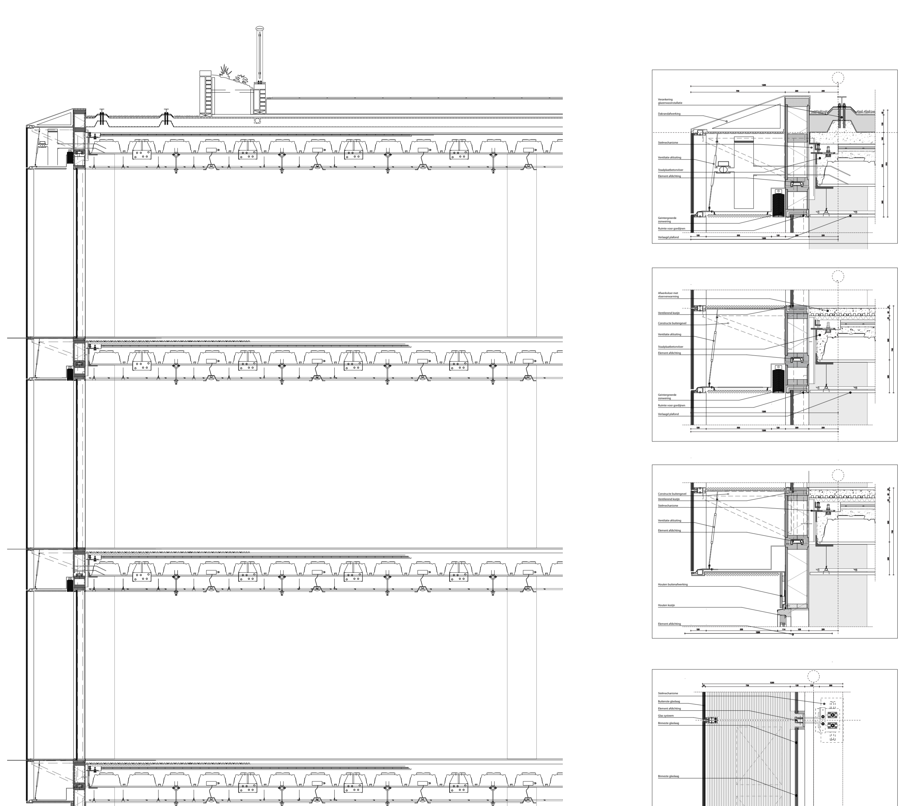
Gevel principedetails 1:20
