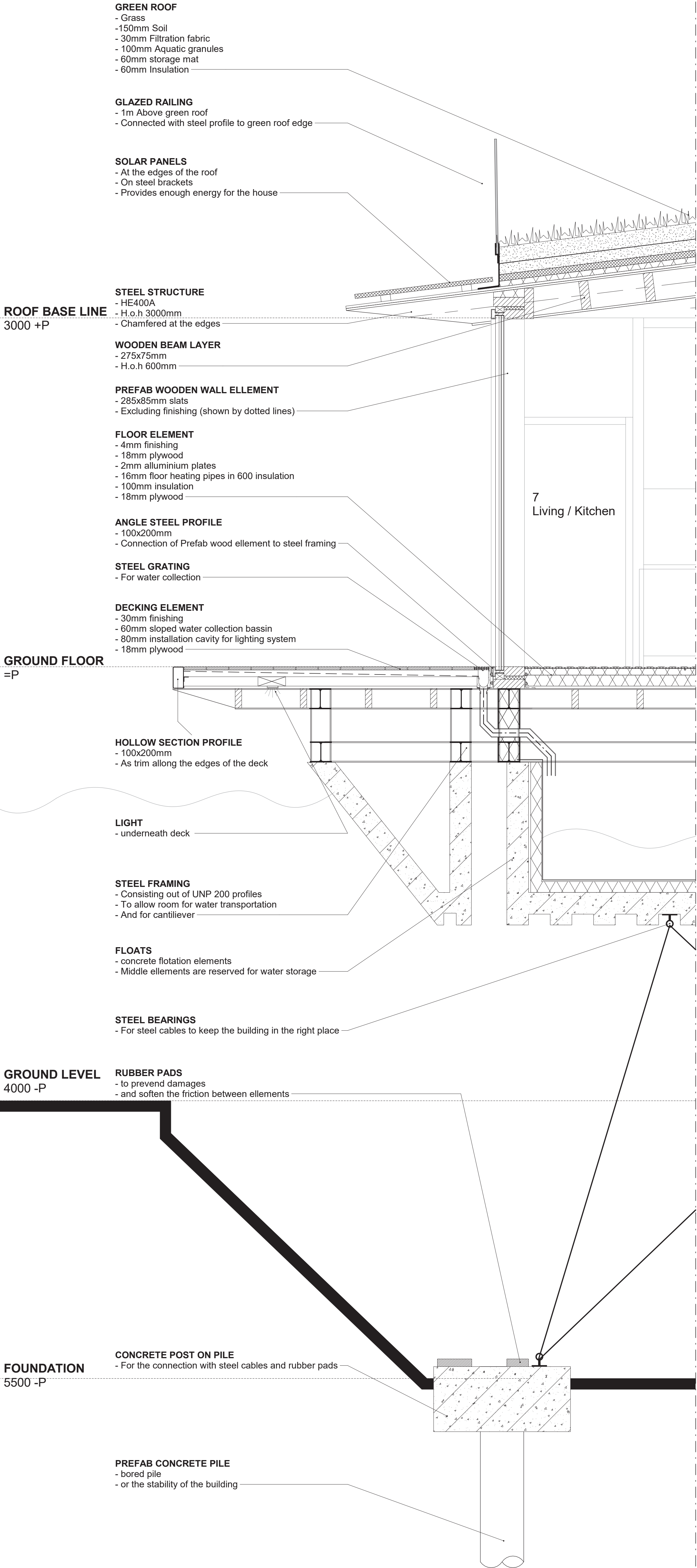
Elevation
