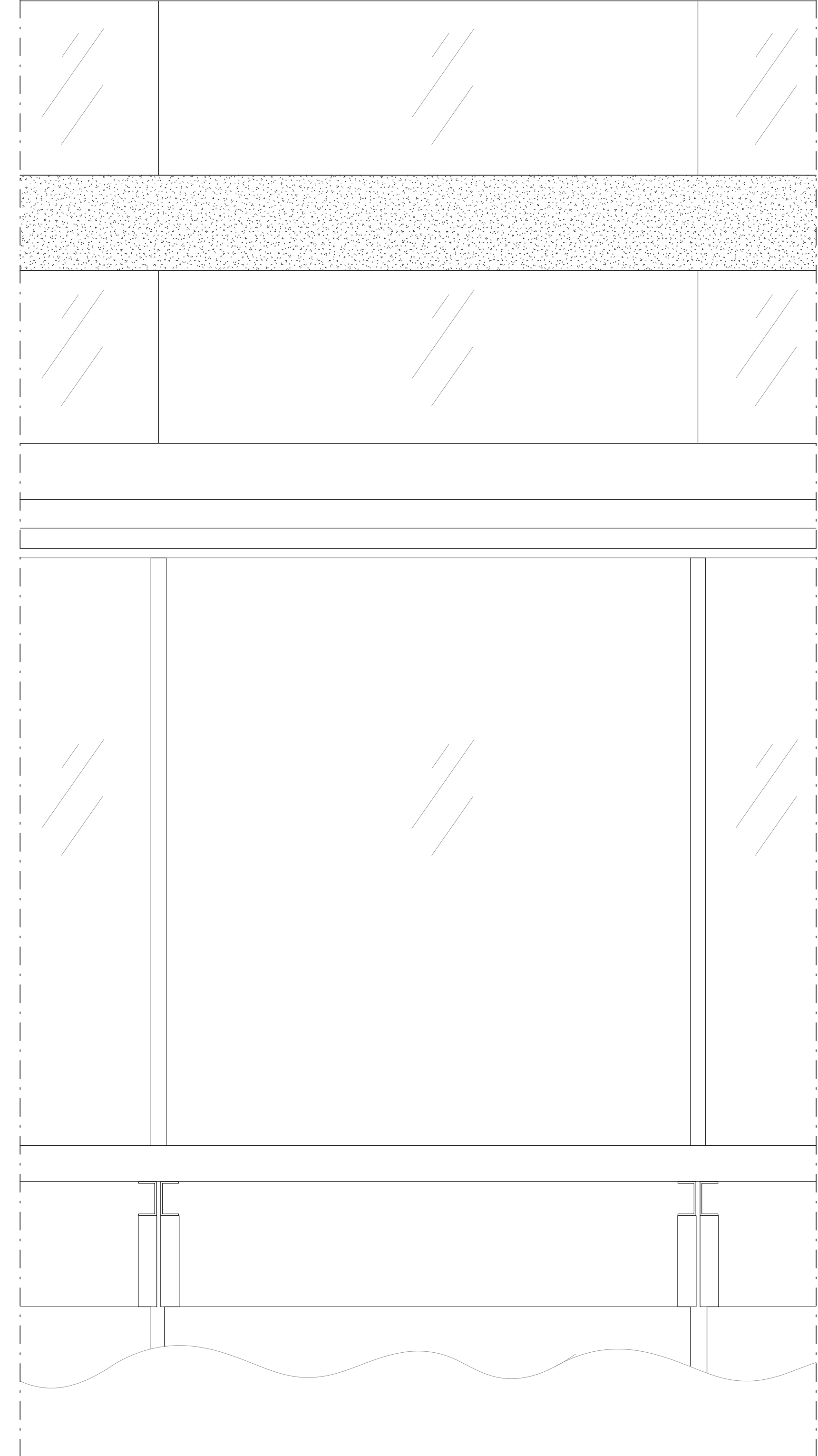
Elevation
