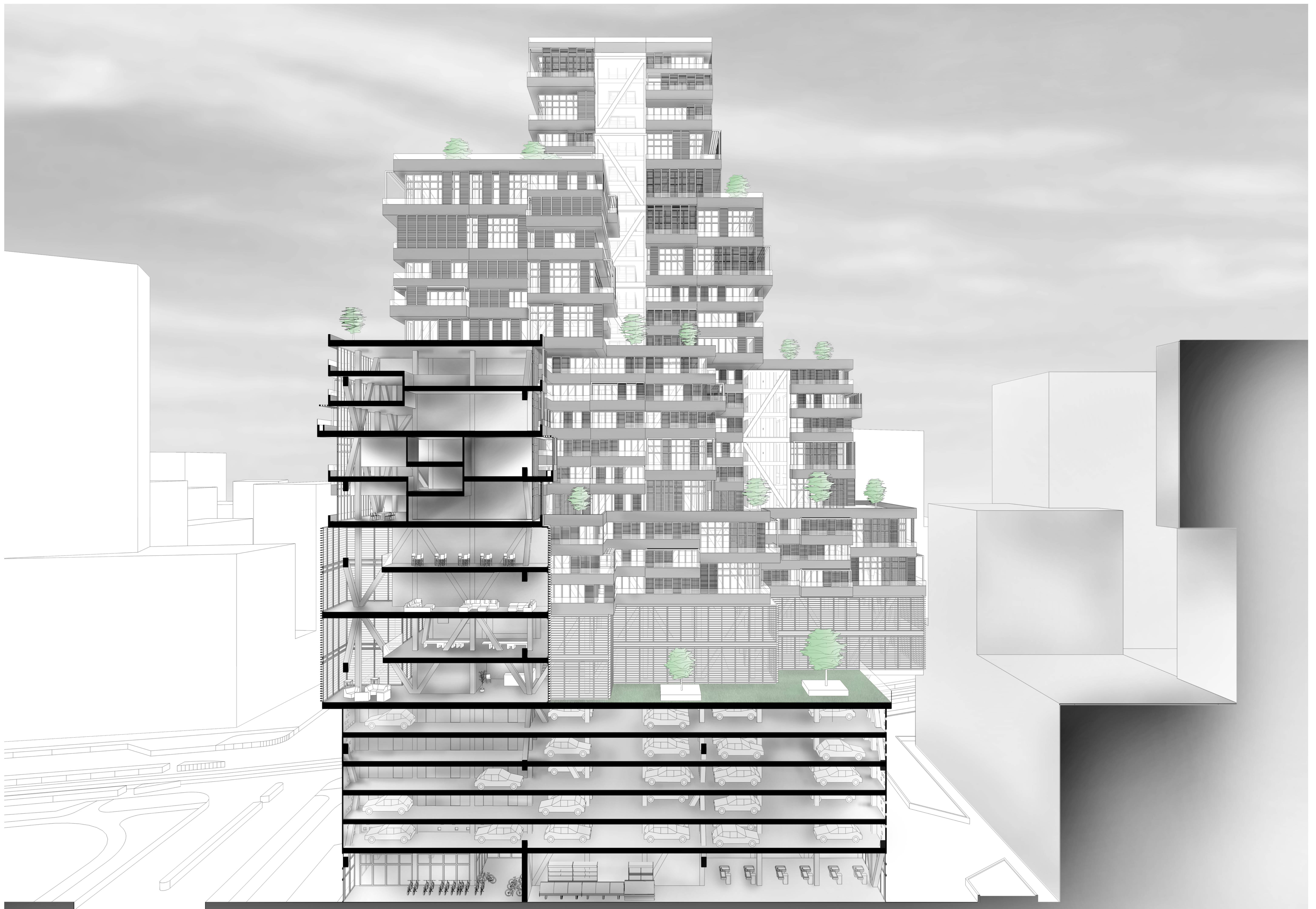
Doorsnede B-B 1:500
