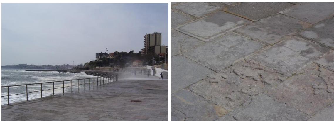
Fig. 10. Achteruitgang van een paar jaar oude kalksteentegels op de esplanade in Cascais waar regelmatig de golven over heen slaan (2010).
