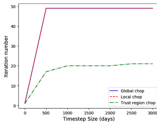
(b) Miscible kernel
