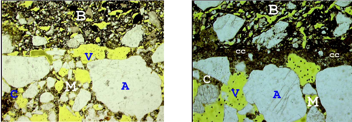
Figuur 2.5 Vergelijking van hechtvlakken. Links: een zwak zuigende steen in contact met een legmortel en rechts. Rechts: een sterk zuigende steen in contact met een legmortel. Het hechtvlak links bevat veel holtes, doordat er nauwelijks vachttransport van de specie naar de zwakzuigende steen heeft plaatsgevonden (maw uitharding van de mortel bij een hoog vochtgehalte). Het hechtvlak rechts bevat veel fijne cementdeeltjes, die daar terecht gekomen zijn tijdens het transport van vocht vanuit de specie naar de sterk zuigende steen; dit gebeurde direct na vermetelsing
