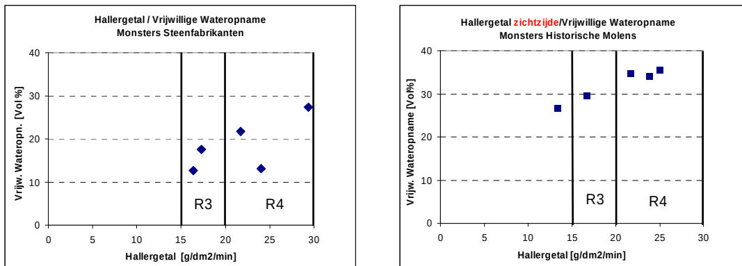
Figuur 5.1. Vergelijking van Hallergetalwaarden en vrijwillige wateropnamen van Monsters Steenfabrieken en Monsters Historische Molens
