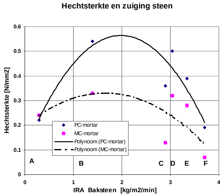
Figuur 2.6 Voor portland cement en metselcement mortels geldt dat de hoogste hechtsterkte wordt bereikt bij stenen met een Hallergetal van 15-25 gr/dm 2 /min (IRA: 1.5-2.5 kg/m 2 /min)
