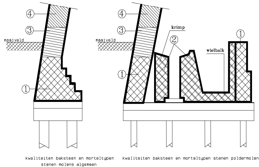
Figuur 2.7 Typen metselwerk (voor betekenis cijfers zie tabel 1)
