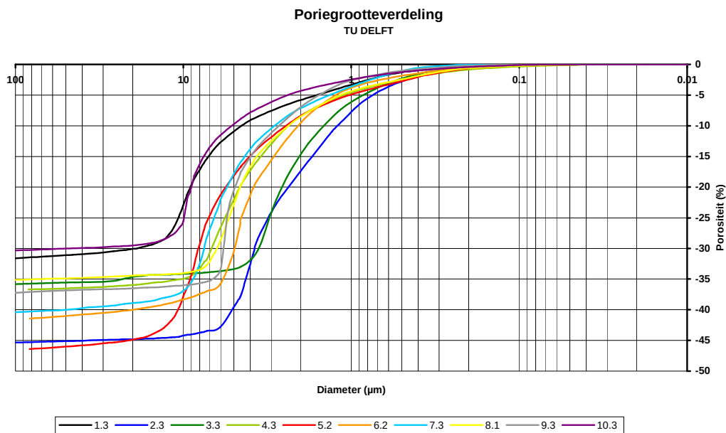
Figuur 3.1. Poriegrootteverdeling van de verschillende monsters ( de getallen verwijzen naar de monsters; bijv. 4.3: aeolus, monster 3, zie verder par. 3.1 monstername)
