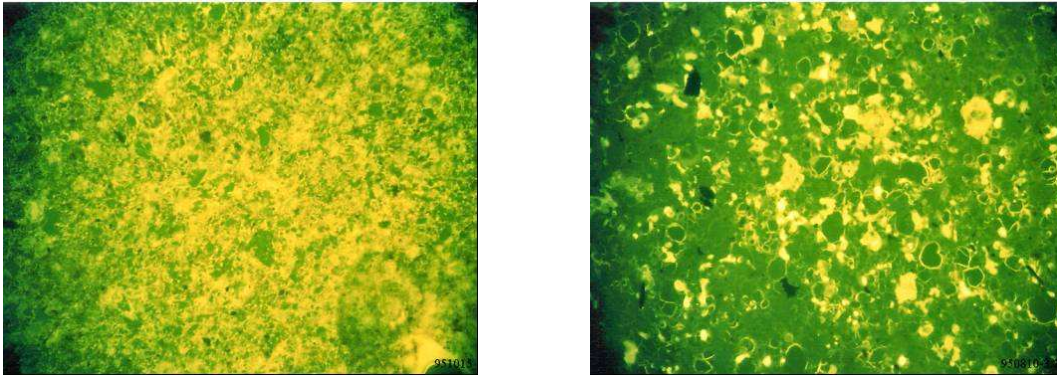
Figuur 2.1 Twee fuorescentie-microfoto's van bakstenen: wit geeft porositeit aan en groen is vaste stof. Links: het sterk verbonden capillair netwerk en een grote opslagcapaciteit van sterk zuigende baksteen (rood); Rechts: geïsoleerde poriën en een geringe opslagcapaciteit van een zwak-zuigende baksteen (klinker) (Rockview, Amsterdam)
