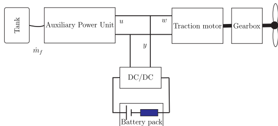
Fig. 1. Powertrain diagram
