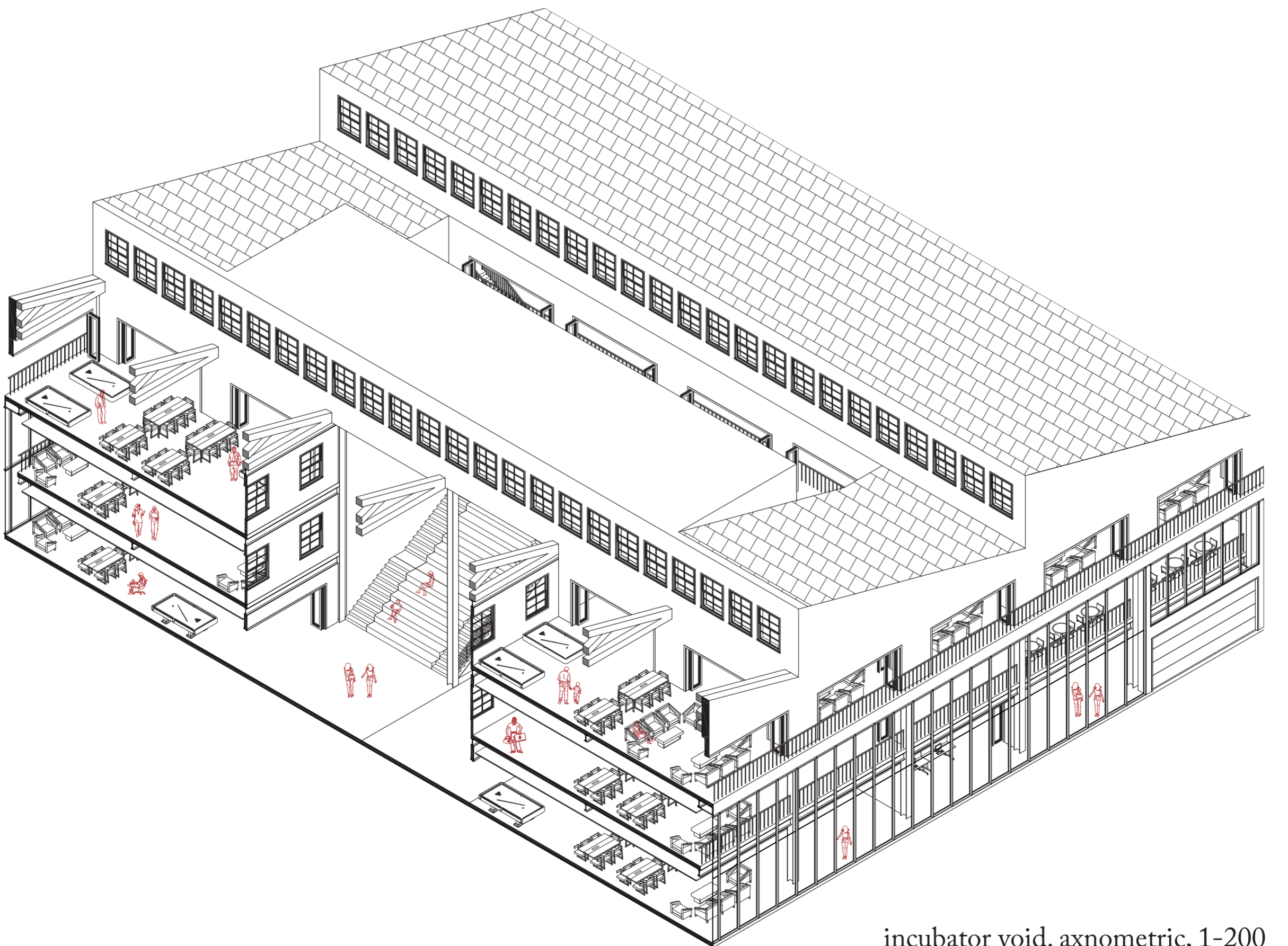
public void. axonometric, 1-200
