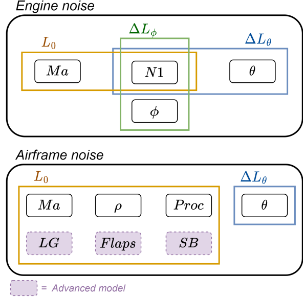
Fig. 2 sonAIR input parameters
