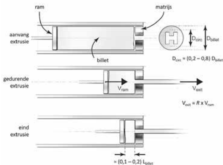
Afbeelding 2 Het extrusieproces schematisch weergegeven.
