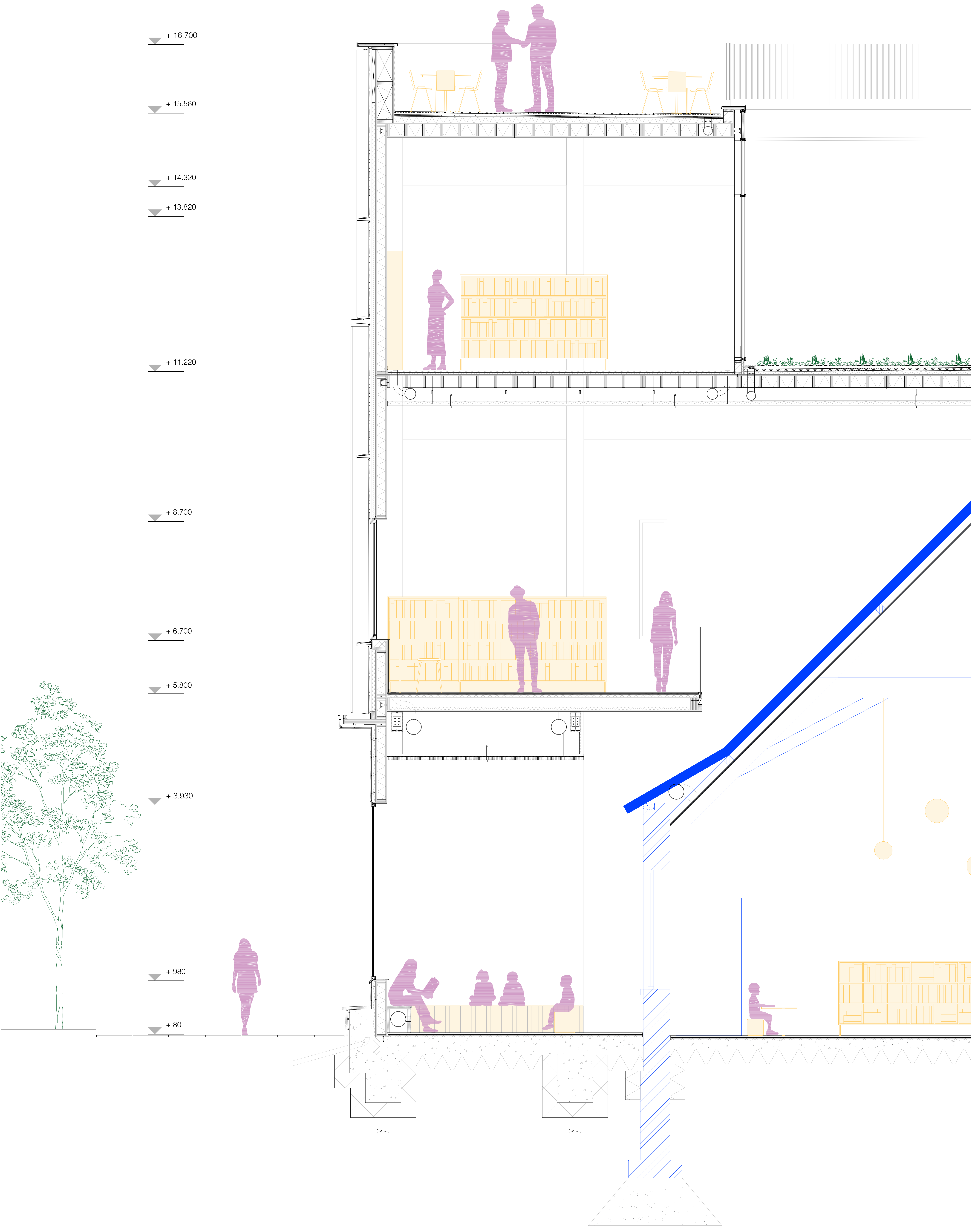
Section 1 : 20
