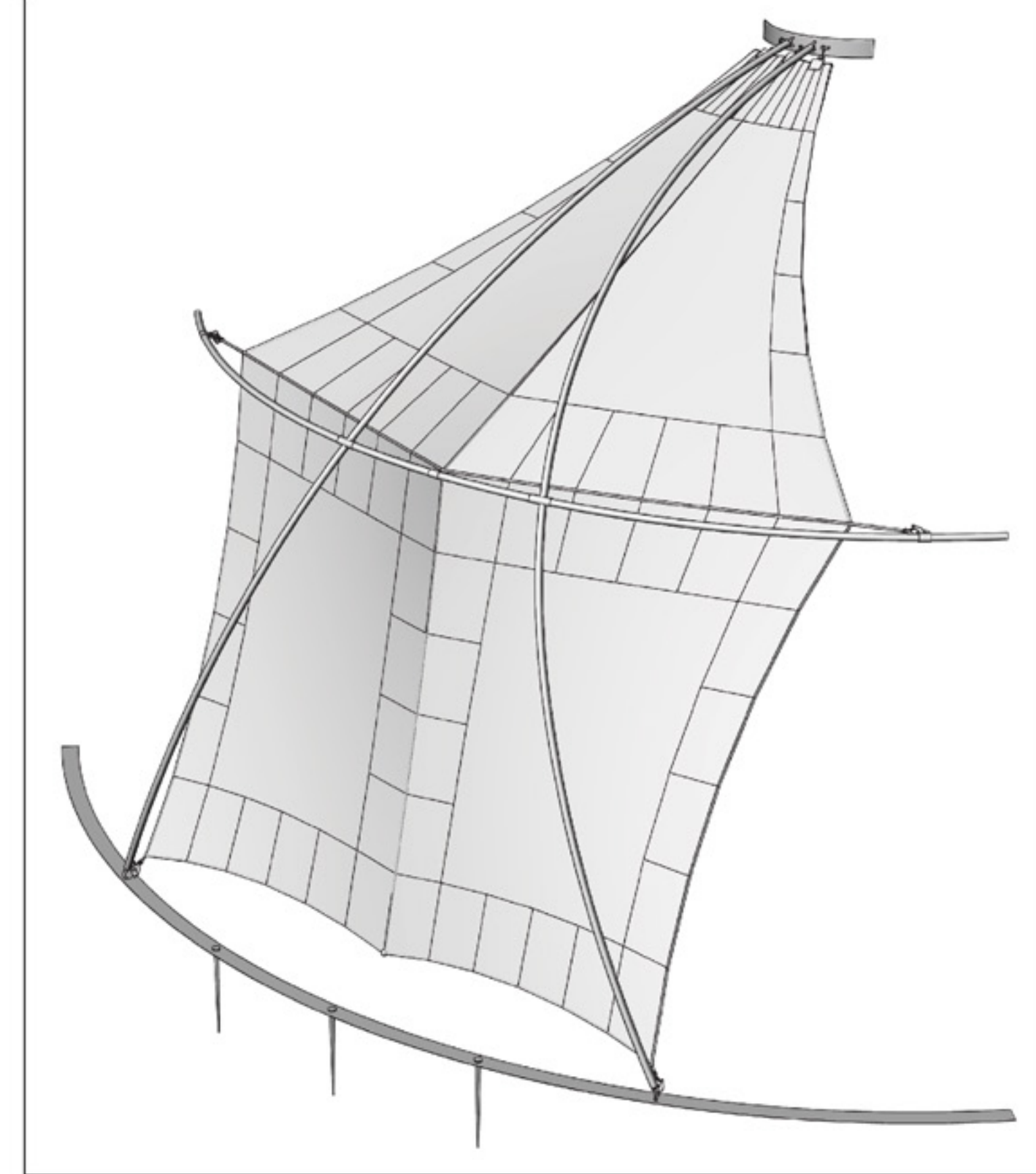
Het Klimbos | Detail B, C
