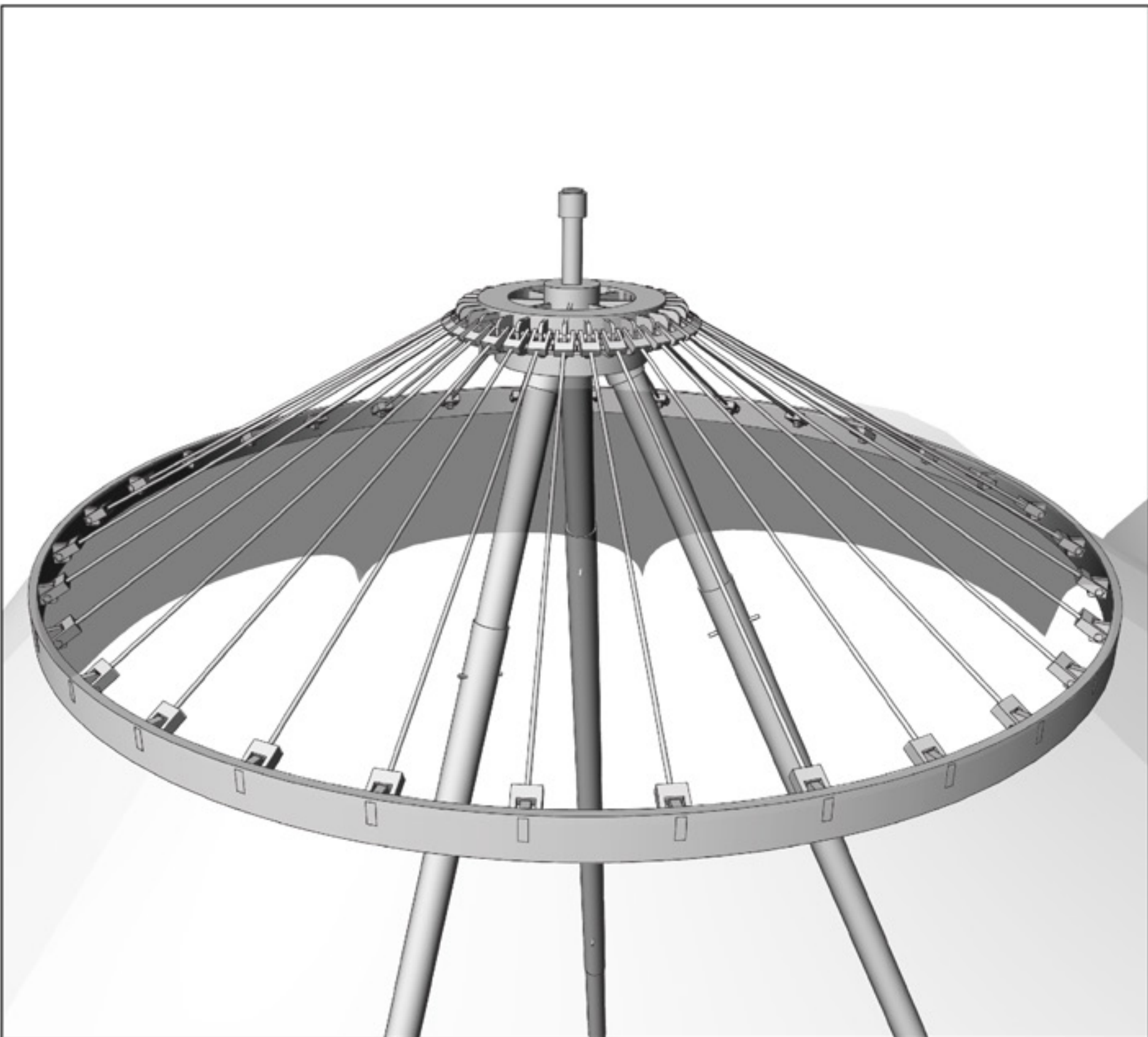
De Kampeertent | Detail D | 1:50
