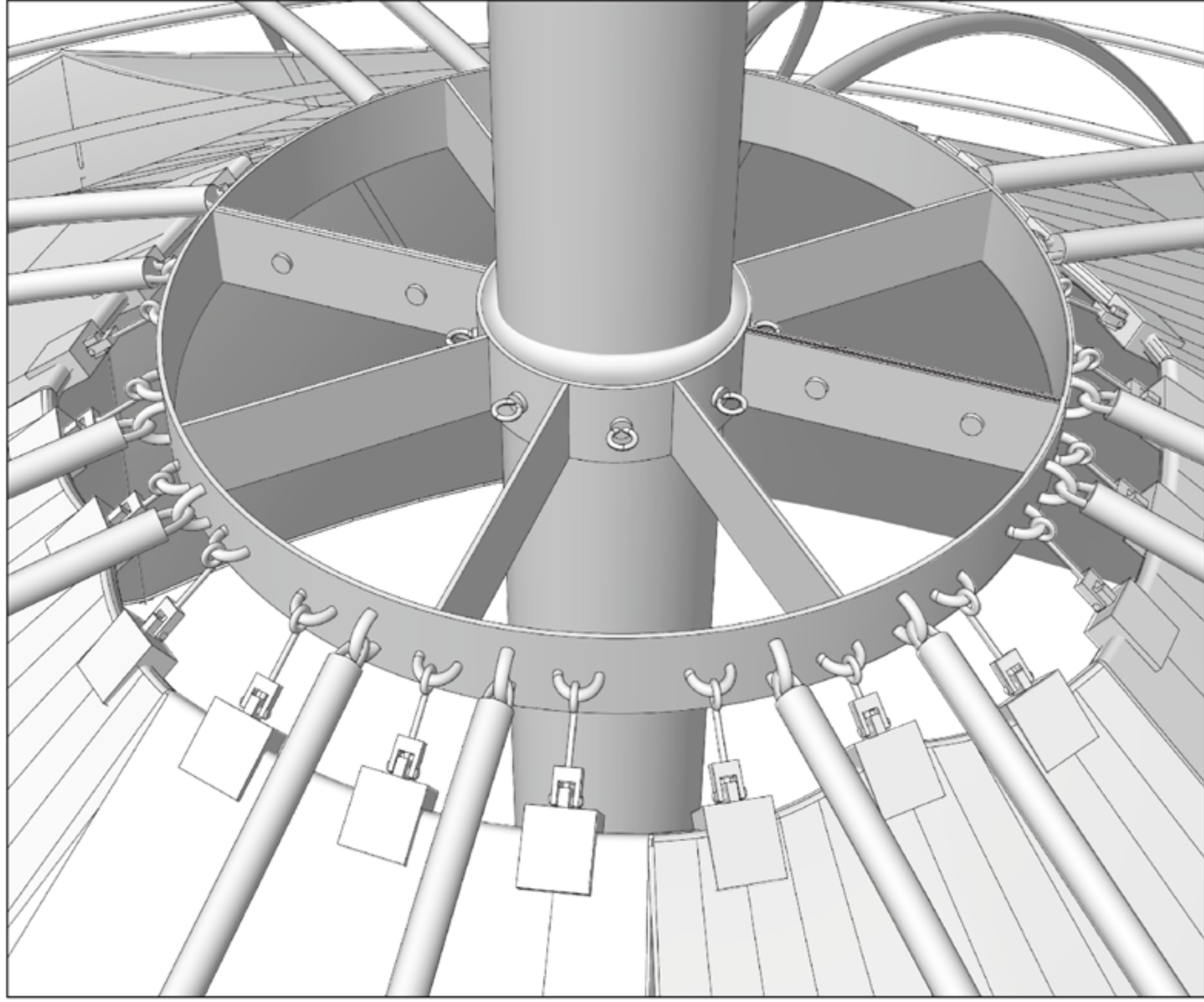
Het Klimbos | Detail A | 1:200
