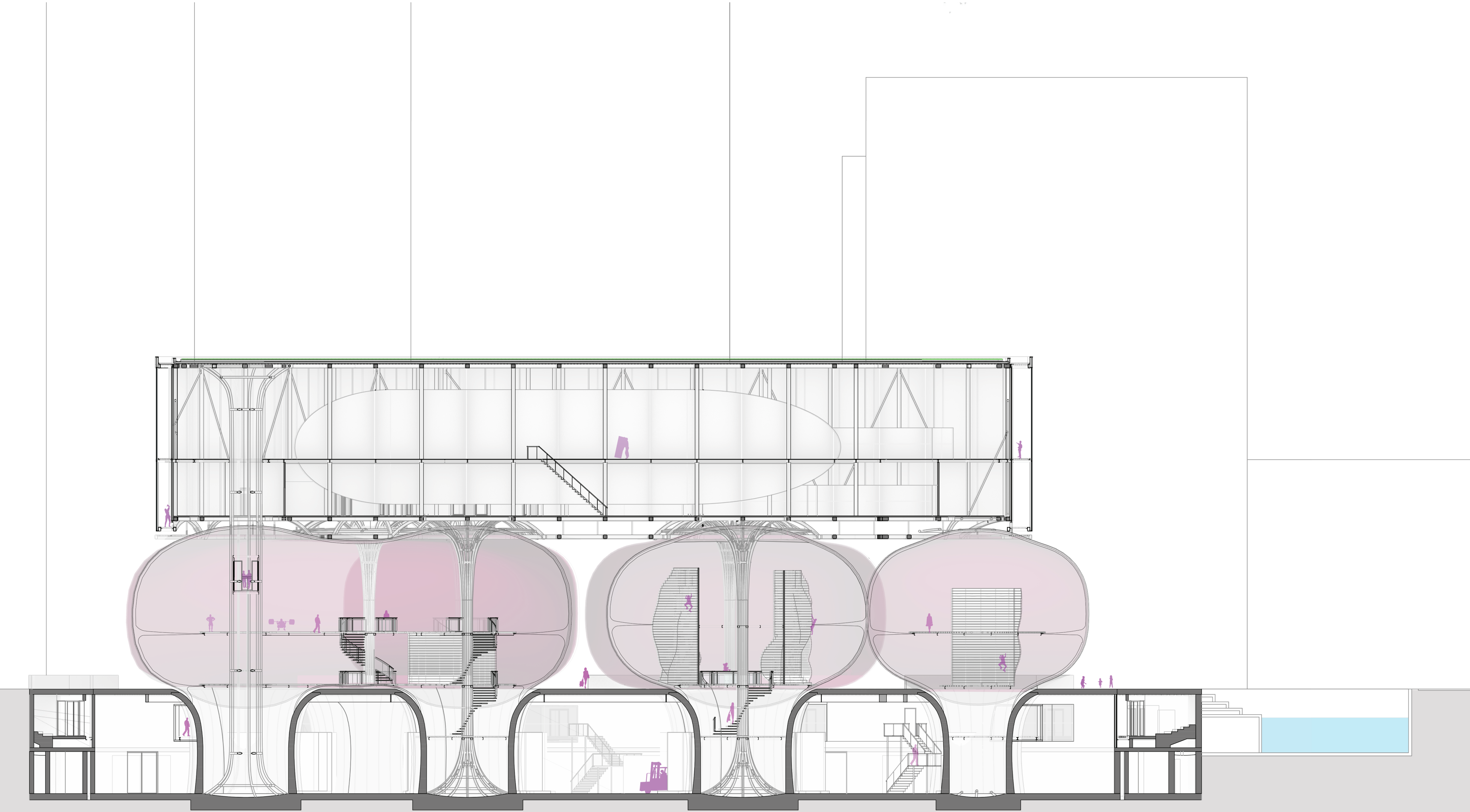
Section A-A' 1:200
