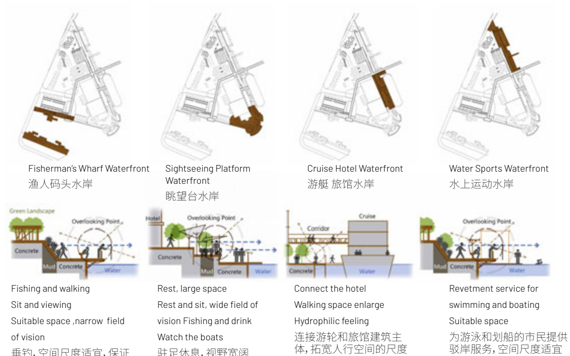
FIG. 2.64 Local Node Perspective 局部节点透视
