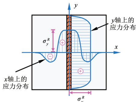
图3 平行焊缝方向残余应力分布
