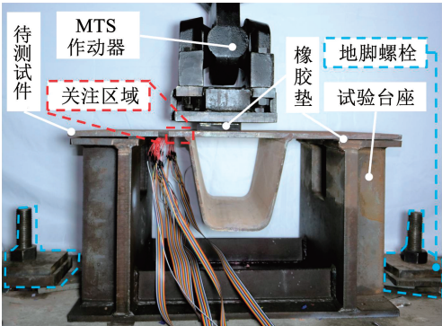
图 7 模型加载
