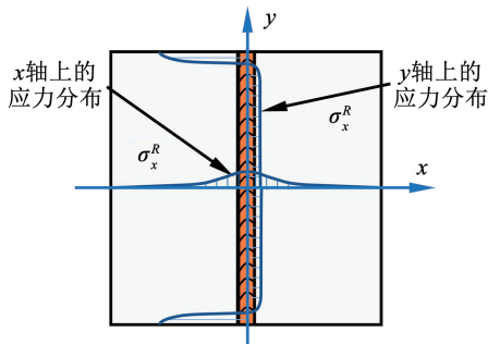
图2 垂直焊缝方向残余应力分布
