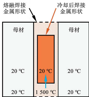
图1 焊接残余应力形成原理
