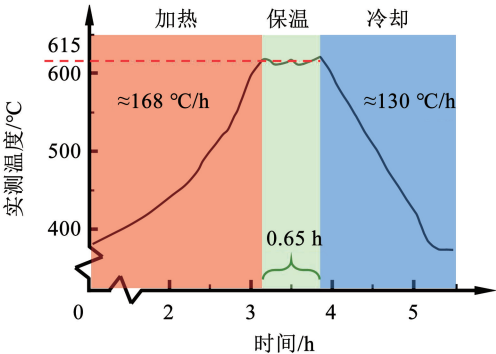
图 6 实测钢桥面温度与时间关系曲线
