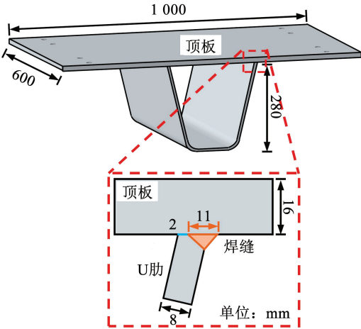
图 4 试验模型与局部构造
