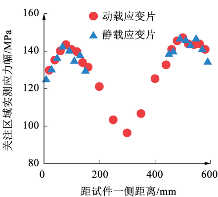
图 12 各测点荷载作用下应力幅
