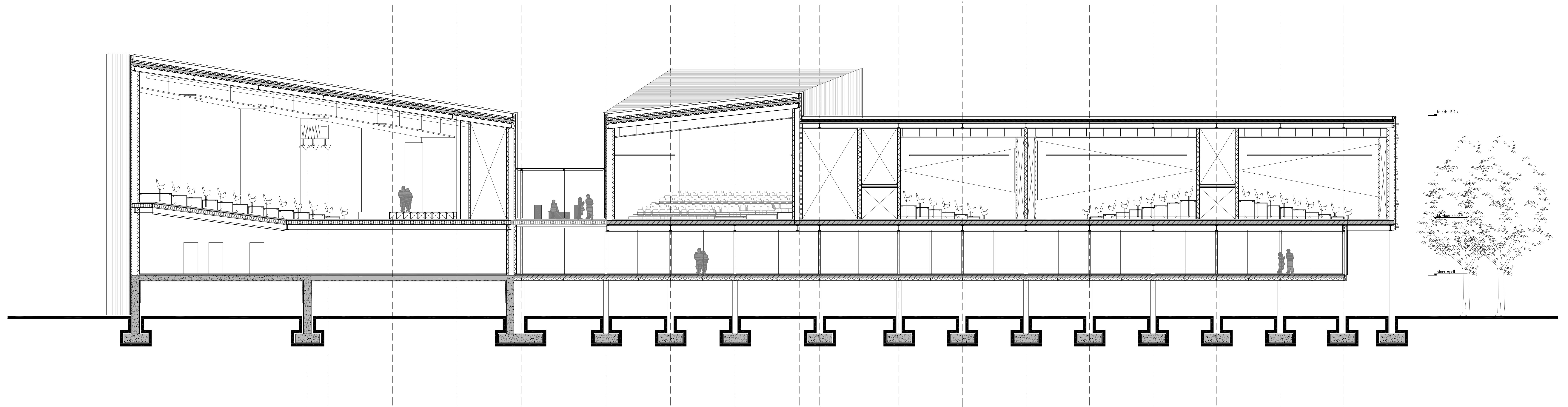
_Langsdoorsnede (1:100)
