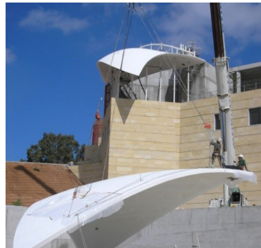
FIG. 7.17 Hijzen van de complete schaal in Tel Aviv
