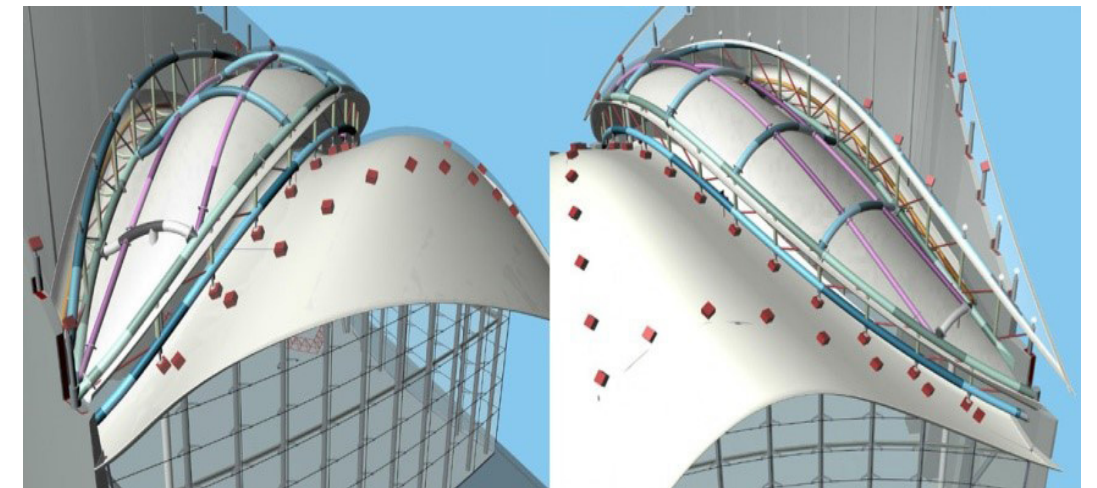
FIG. 7.11 Compositie van element-engineeringen van de central body van de Great Hall van Rabin Center, Octatube
