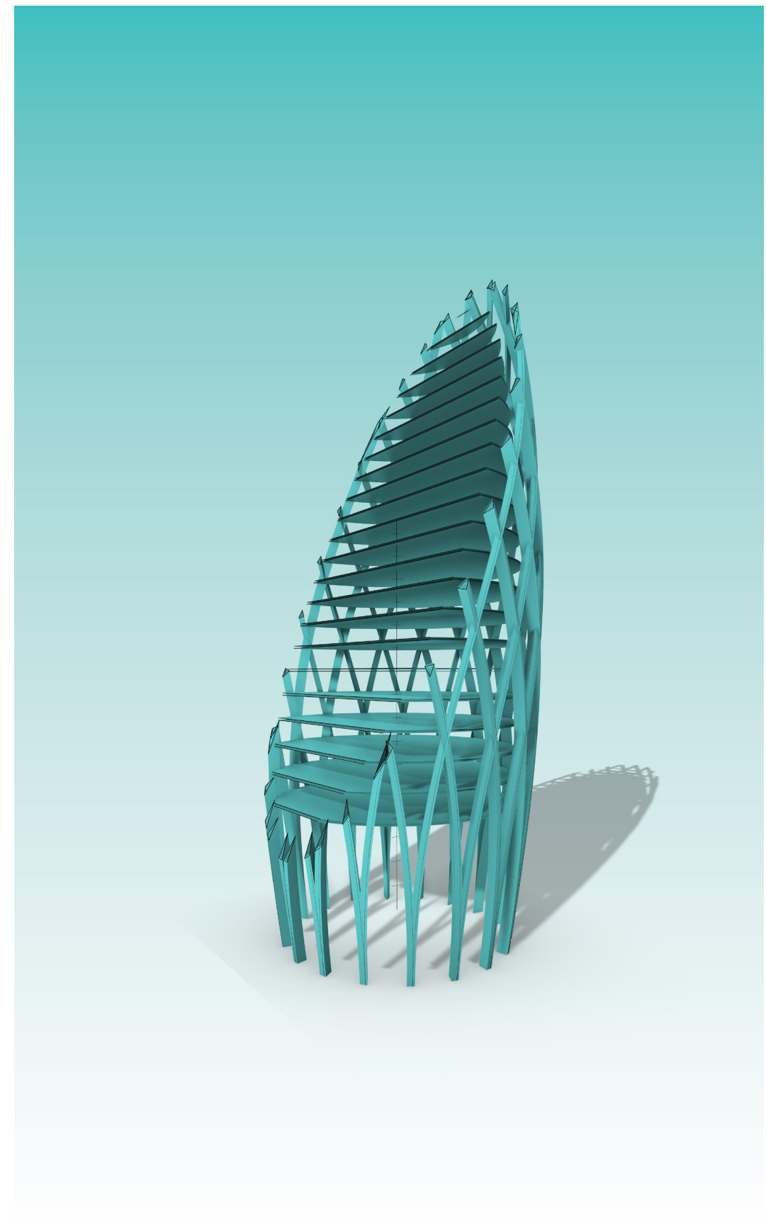
FIG. 3.19 3D structuur Swiss Re met clipping plane
