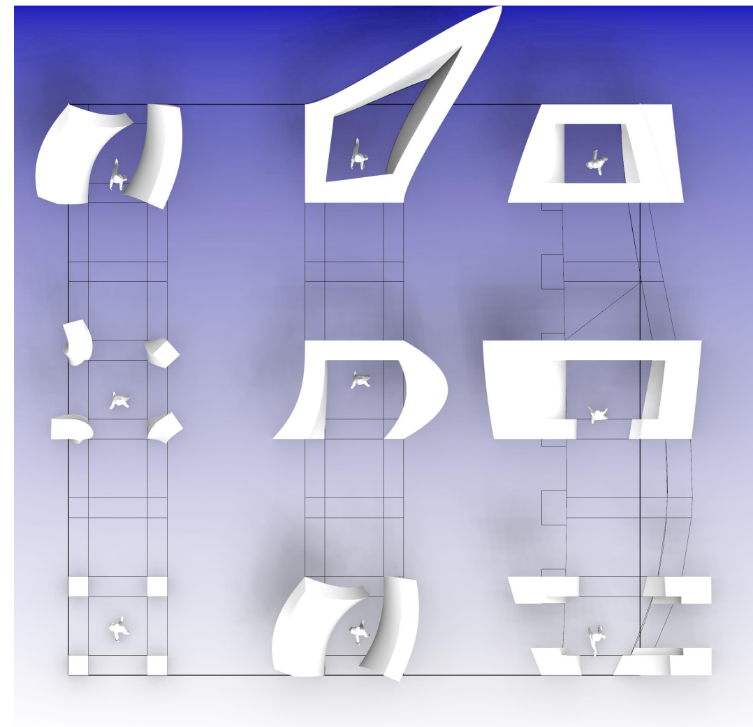
FIG. 4.28 Vrijevorm ruimtevorming
