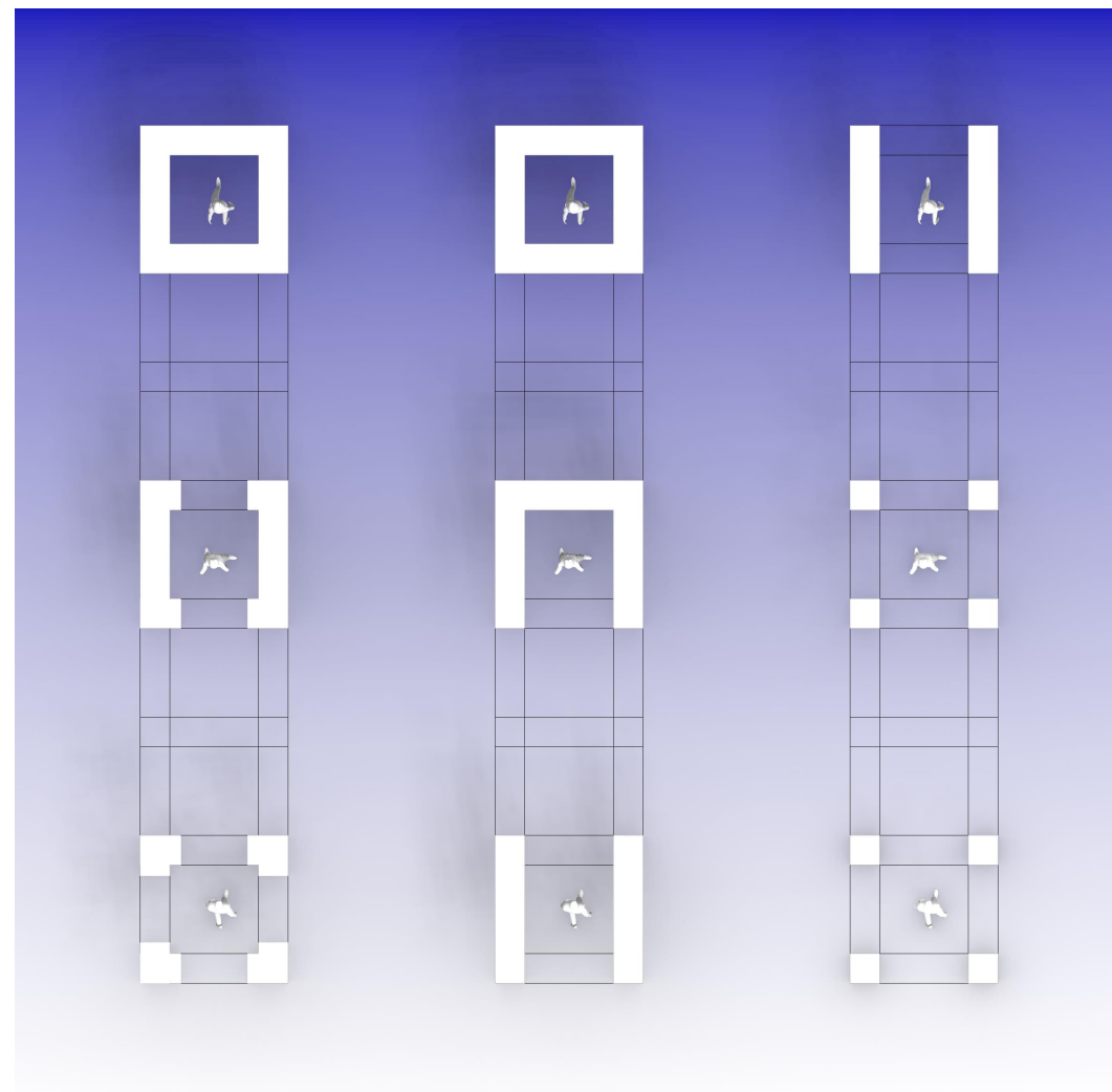
FIG. 4.27 Klassieke ruimtevorming
