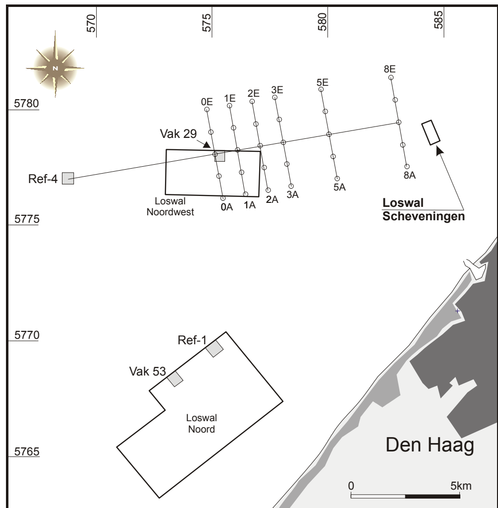
Figuur 11-1 Monitoringslocaties ecotoxicologische metingen
