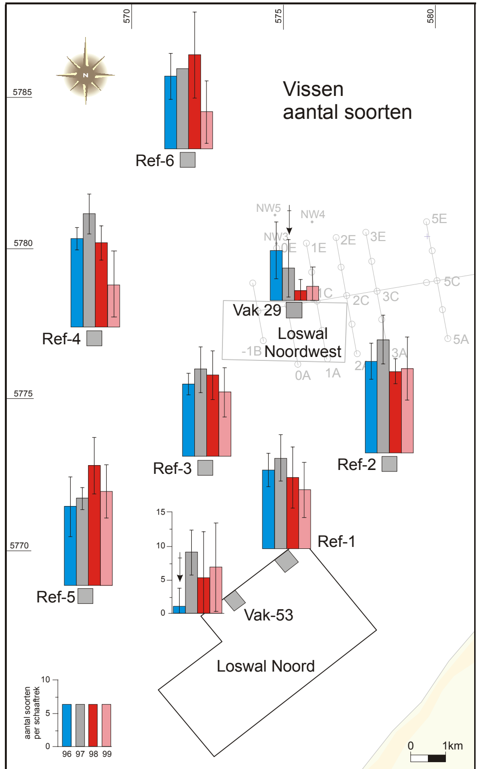
Loswal Noord en Noordwest en referentielocaties in 1996 tot en met 1999. Het gemiddeld aantal soorten vissen per schaaftrek met 95% betrouwbaarheidsgrenzen. Pijlen duiden op storting van baggerspecie. (NIOZ)
