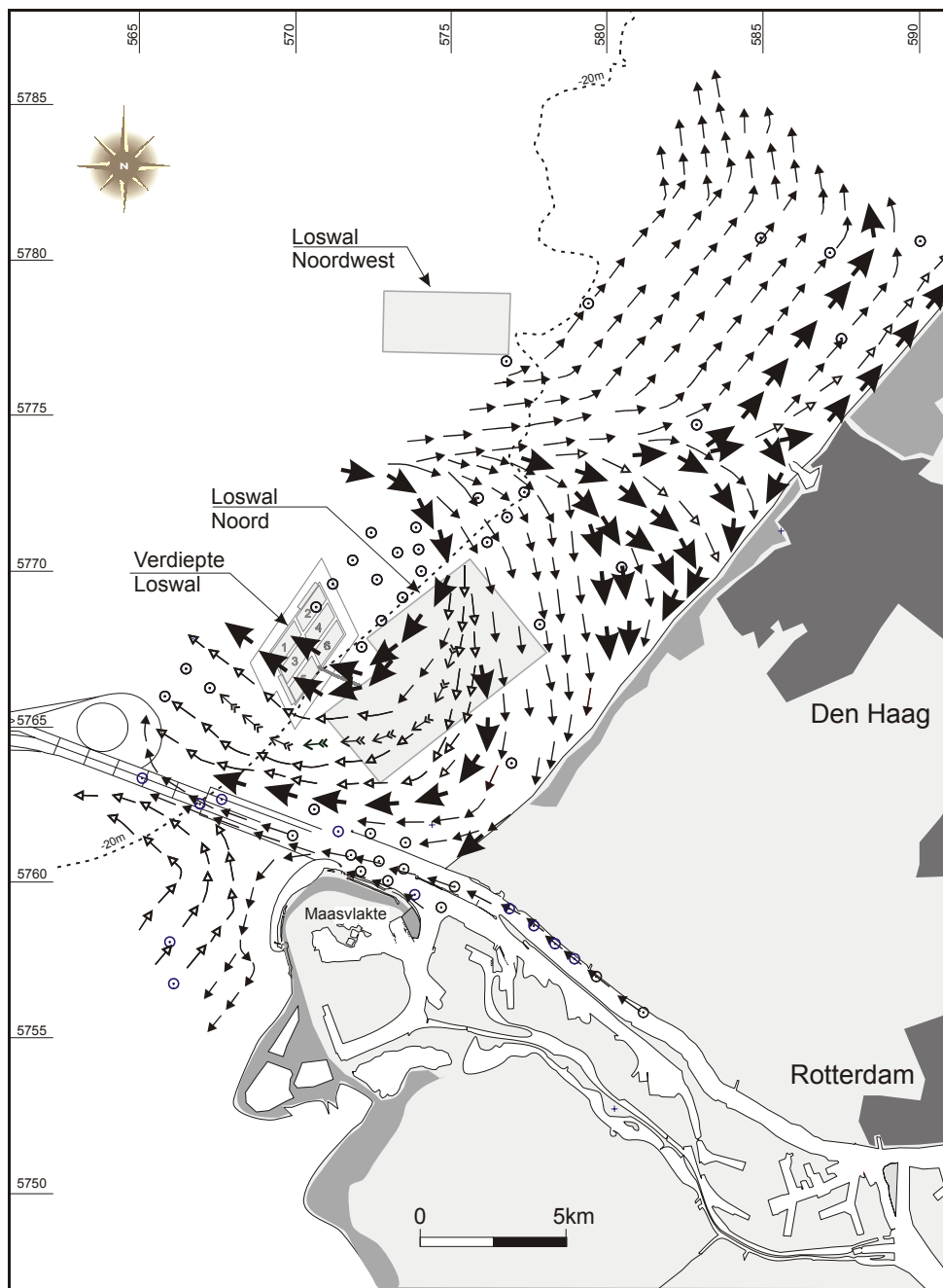
Figuur 4-4 Patroon van netto zandtransport langs de Zuid-Hollandse kust
