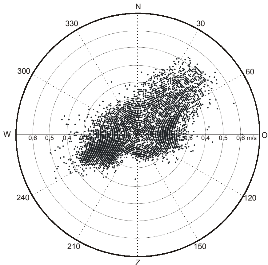
Figuur 8-1 Stroomrichting en stroomsnelheid op Loswal Noordwest
