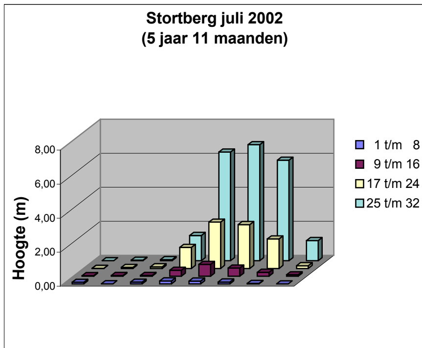
Figuur 6-3 Vorm van de stortberg op Loswal Noordwest
