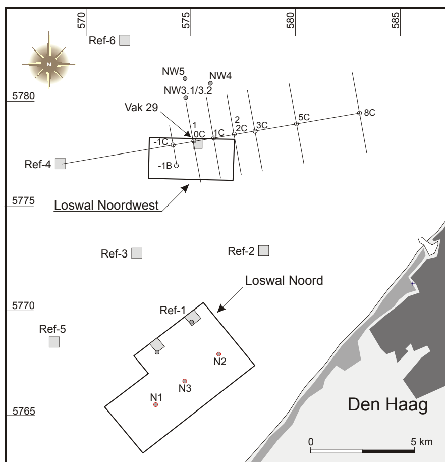
Figuur 12-1 Monitoringslocaties van Macrocenthos
