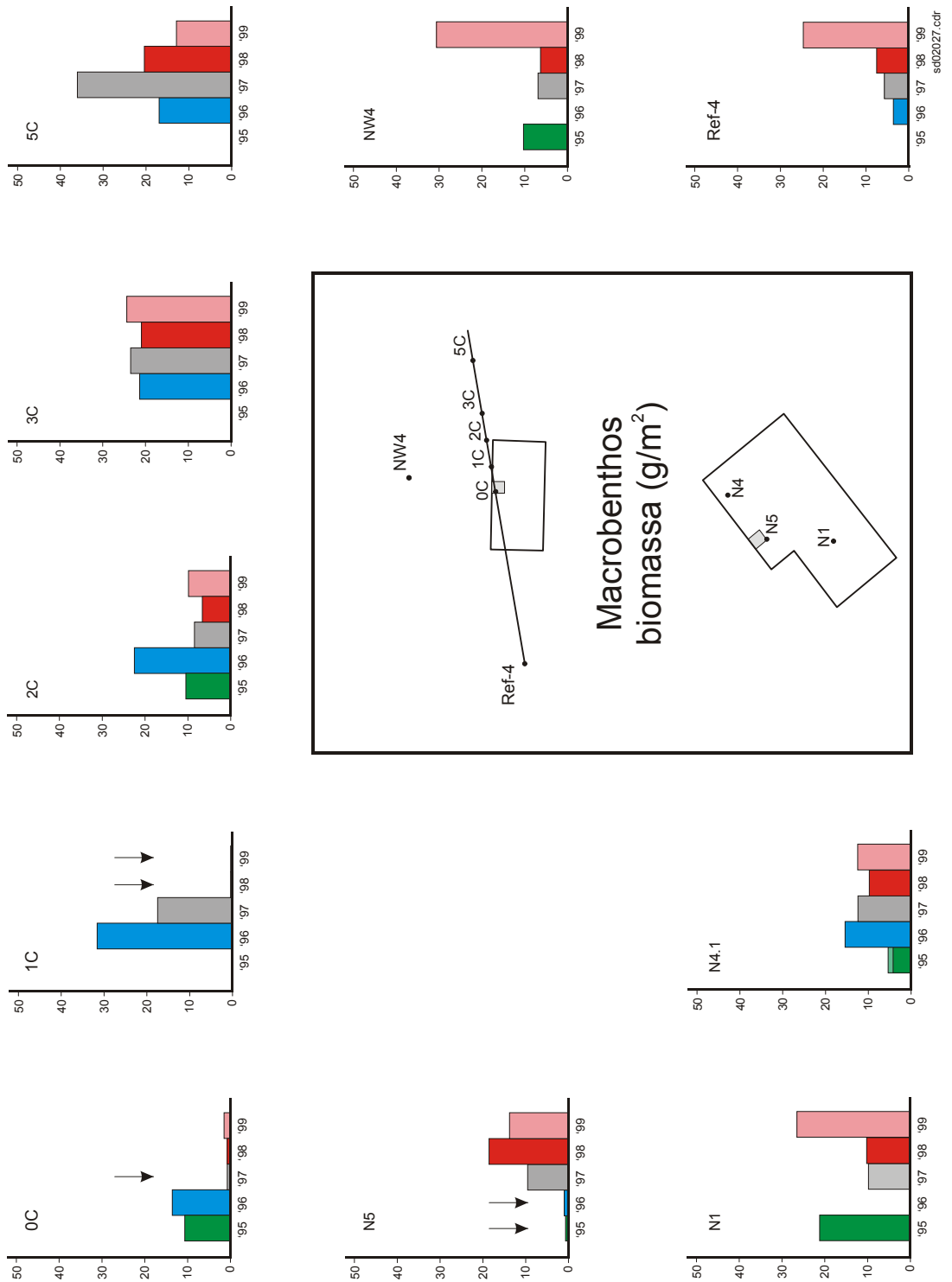
Figuur 12-6 Biomassa Macrobenthos
