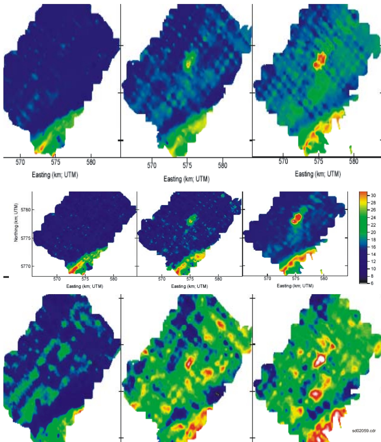
Figuur 6-9 Verdeling natuurlijke radioactiviteit rondom Loswal Noordwest
