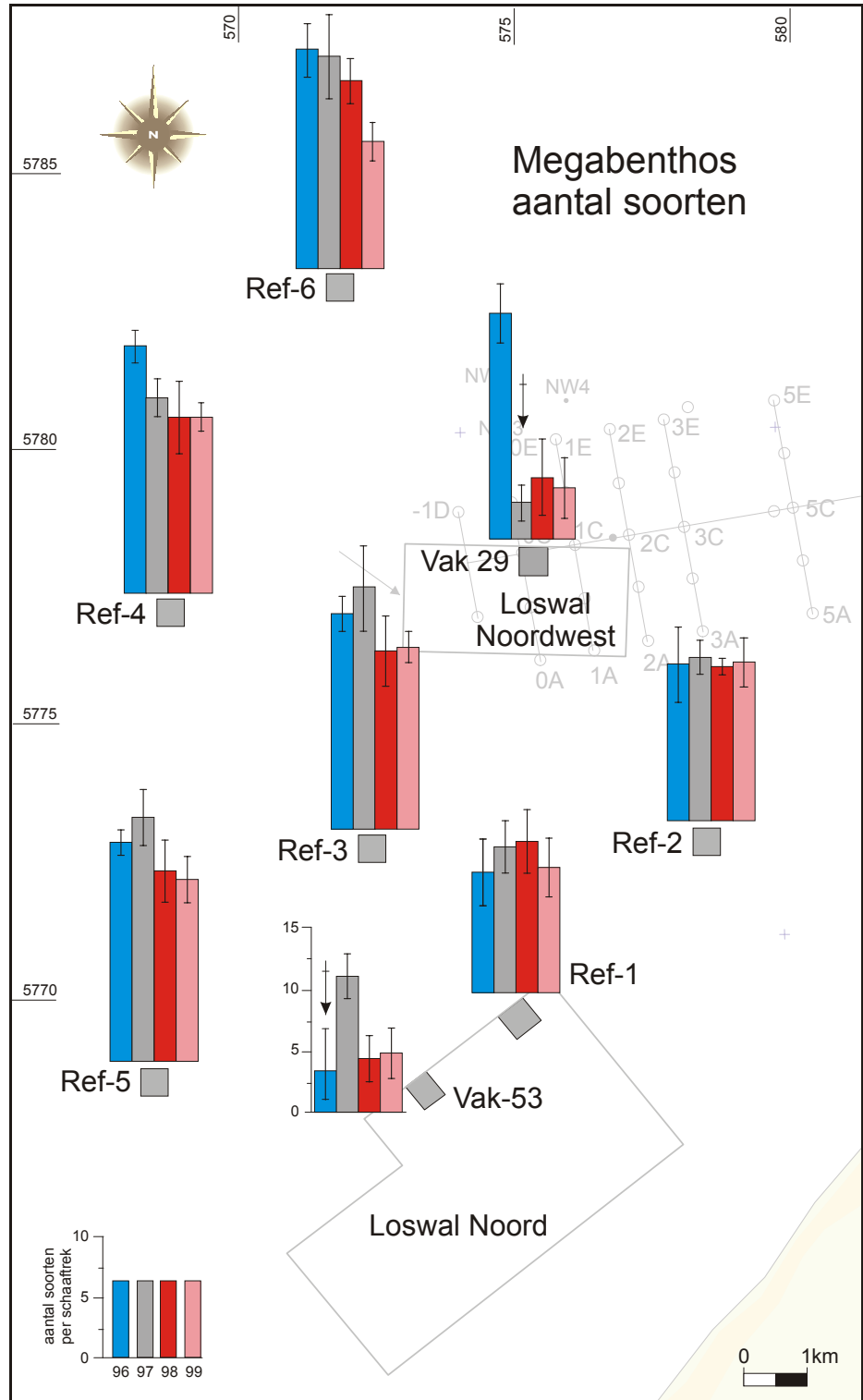
Figuur 12-9 Aantal soorten Megabenthos 1996 t/m 1999
