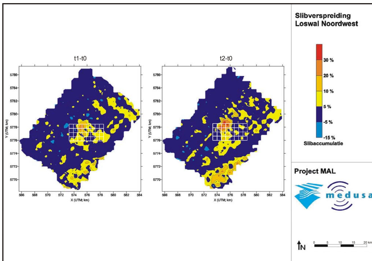
Figuur 6-12 Achtergebleven slib < 63 μm rondom Loswal Noordwest
