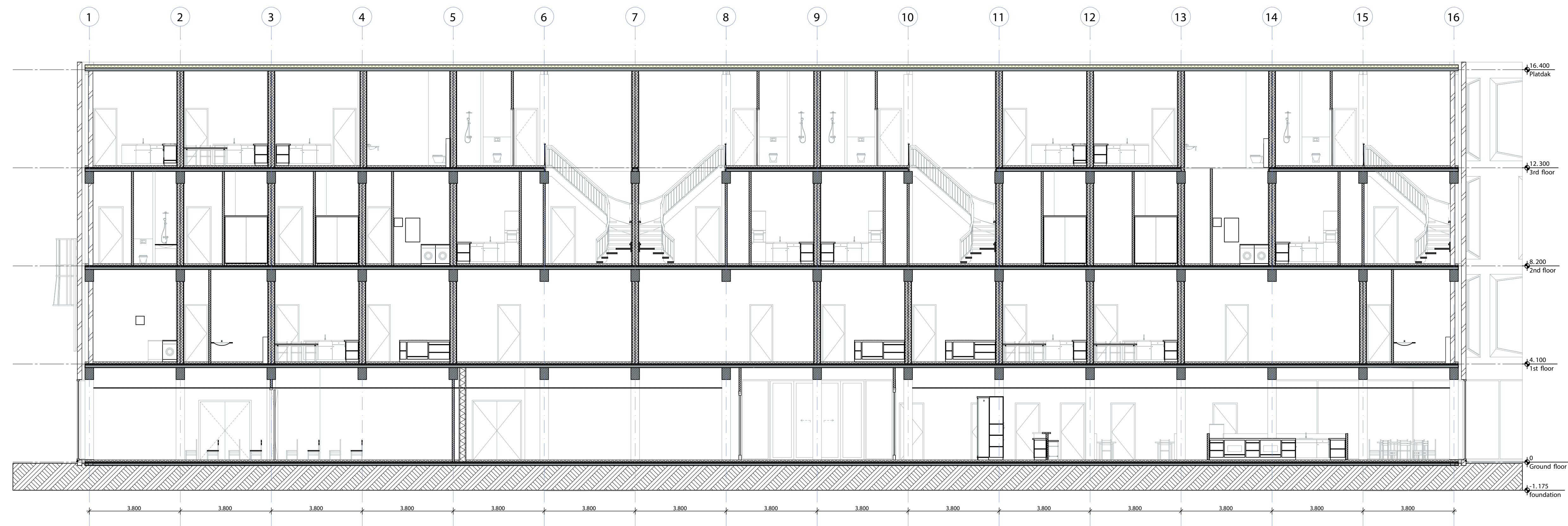
Longitudinal section A - A
